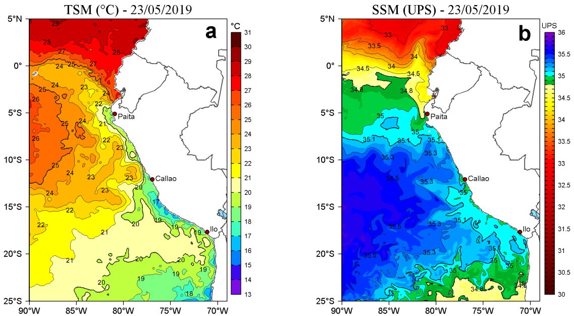
Figura 2. a) Temperatura superficial del mar (TSM, °C) y b) Salinidad superficial del mar (SSM, UPS), para el 23 de mayo de 2019. Datos: OSTIA-UKMO-L4-GLOB-v2.0 (UK Met Office, 2012; Donlon et al, 2012) disponible en https://podaac.jpl.nasa.gov/dataset/OSTIA-UKMO-L4-GLOB-v2.0 para (a) y Hybrid Coordinate Ocean Model v. GOF3.1 (HYCOM; Halliwell et al., 1998; 2000; Bleck, 2001) para (b). Procesamiento: LHF/AFIOF/DGIOCC/IMARPE.
