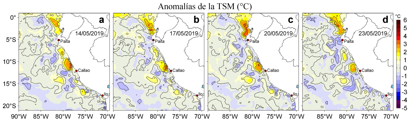
Figura 3. Anomalías de la temperatura superficial del mar (TSM, °C) para los días: a) 14, b) 17, c) 20 y d) 23 de mayo de 2019. Las anomalías se calcularon respecto de la climatología para el periodo 2007-2016. Datos: OSTIA-UKMO-L4-GLOB-v2.0 (UK Met Office, 2012; Donlon et al, 2012). Procesamiento: LHF/AFIOF/DGIOCC/IMARPE.
