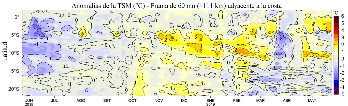
Figura 4. Variación promedio de las anomalías de la temperatura superficial del mar (TSM, °C) para una franja de 60 mn (~111 km) adyacente al litoral peruano para los últimos doce meses al 23 de mayo de 2019. Datos: OSTIA-UKMO-L4-GLOB-v2.0 (UK Met. Office, 2012; Donlon et al, 2012) disponible en https://podaac.jpl.nasa.gov/dataset/OSTIA-UKMO-L4-GLOB-v2.0 . Las anomalías se calcularon con respecto al periodo 2007-2016. Procesamiento: LHF/AFIOF/DGIOCC/IMARPE.
