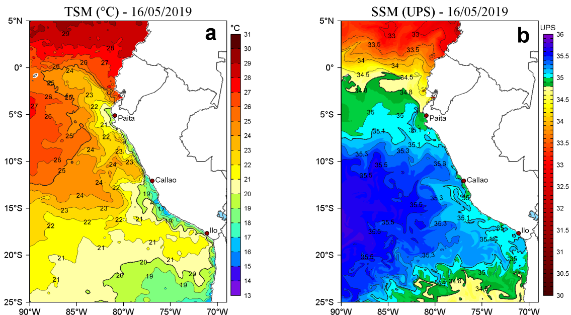
Figura 2. a) Temperatura superficial del mar (TSM, °C) y b) Salinidad superficial del mar (SSM, UPS), para el 16 de mayo de 2019. Datos: OSTIA-UKMO-L4-GLOB-v2.0 (UK Met Office, 2012; Donlon et al, 2012) disponible en https://podaac.jpl.nasa.gov/dataset/OSTIA-UKMO-L4-GLOB-v2.0 para (a) y Hybrid Coordinate Ocean Model v. GOFS 3.1 (HYCOM; Halliwell et al., 1998; 2000; Bleck, 2001) para (b). Procesamiento: LHFM/AFIOF/DGIOCC/IMARPE.
