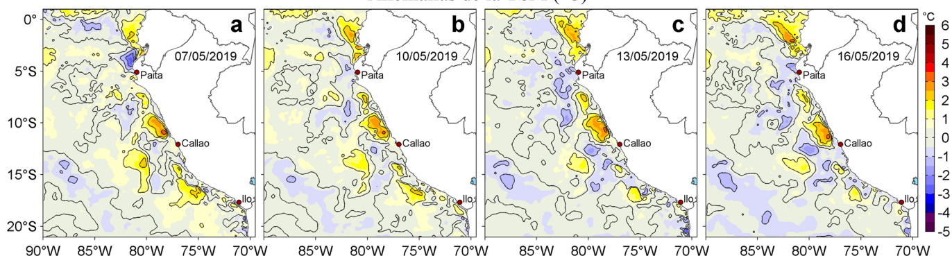
Figura 3. Anomalías de la temperatura superficial del mar (TSM, °C) para los días: a) 07, b) 10, c) 13 y d) 16 de mayo de 2019. Las anomalías se calcularon respecto de la climatología para el periodo 2007-2016. Datos: OSTIA-UKMO-L4-GLOB-v2.0 (UK Met Office, 2012; Donlon et al, 2012). Procesamiento: LHFM/AFIOF/DGIOCC/IMARPE.
