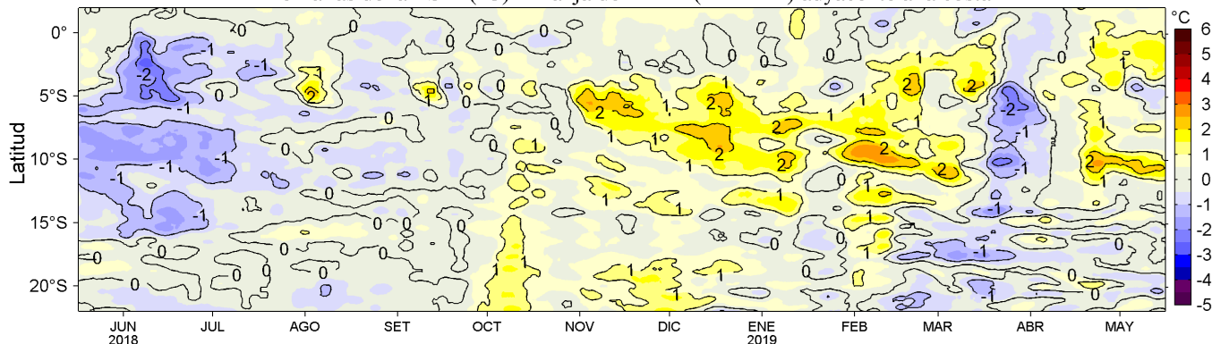
Figura 4. Variación promedio de las anomalías de la temperatura superficial del mar (TSM, °C) para una franja de 60 mn (~111 km) adyacente al litoral peruano para los últimos doce meses al 16 de mayo de 2019. Datos: OSTIA-UKMO-L4-GLOB-v2.0 (UK Met. Office, 2012; Donlon et al, 2012) disponible en https://podaac.jpl.nasa.gov/dataset/OSTIA-UKMO-L4-GLOB-v2.0 . Las anomalías se calcularon con respecto al periodo 2007-2016. Procesamiento: LHFM/AFIOF/DGIOCC/IMARPE.
