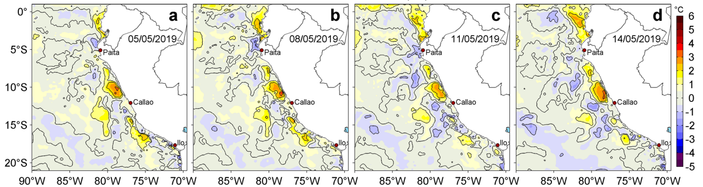
Figura 3. Anomalías de la temperatura superficial del mar (TSM, °C) para los días: a) 05, b) 08, c) 11 y d) 14 de mayo de 2019. Las anomalías se calcularon respecto de la climatología para el periodo 2007-2016. Datos: OSTIA-UKMO-L4-GLOB-v2.0 (UK Met Office, 2012; Donlon et al, 2012). Procesamiento: LHFM/AFIOF/DGIOCC/IMARPE.
