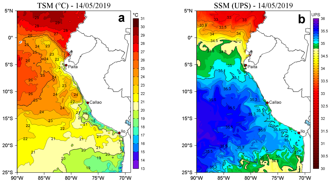
Figura 2. a) Temperatura superficial del mar (TSM, °C) y b) Salinidad superficial del mar (SSM, UPS), para el 14 de mayo de 2019. Datos: OSTIA-UKMO-L4-GLOB-v2.0 (UK Met Office, 2012; Donlon et al, 2012) disponible en https://podaac.jpl.nasa.gov/dataset/OSTIA-UKMO-L4-GLOB-v2.0 para (a) y Hybrid Coordinate Ocean Model v. GOFS 3.1 (HYCOM; Halliwell et al., 1998; 2000; Bleck, 2001) para (b). Procesamiento: LHFM/AFIOF/DGIOCC/IMARPE.
