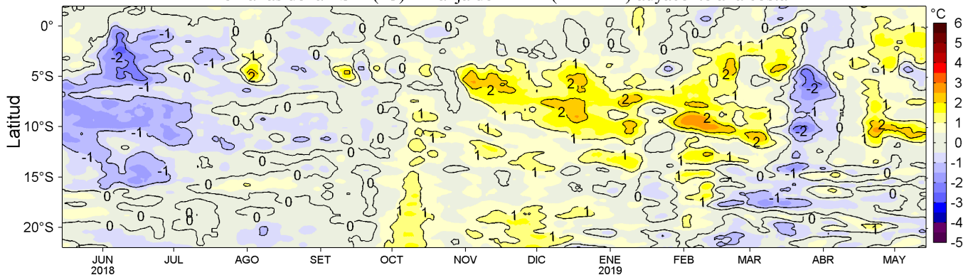
Figura 4. Variación promedio de las anomalías de la temperatura superficial del mar (TSM, °C) para una franja de 60 mn (~111 km) adyacente al litoral peruano para los últimos doce meses al 14 de mayo de 2019. Datos: OSTIA-UKMO-L4-GLOB-v2.0 (UK Met. Office, 2012; Donlon et al, 2012) disponible en https://podaac.jpl.nasa.gov/dataset/OSTIA-UKMO-L4-GLOB-v2.0 . Las anomalías se calcularon con respecto al periodo 2007-2016. Procesamiento: LHFM/AFIOF/DGIOCC/IMARPE.
