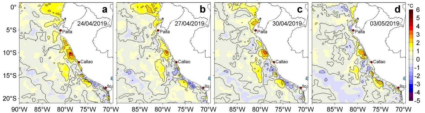
Figura 3. Anomalías de la temperatura superficial del mar (TSM, °C) para los días: a) 24, b) 27 y c) 30 de abril y d) 03 de mayo de 2019. Las anomalías se calcularon respecto de la climatología para el periodo 2007-2016. Datos: OSTIA-UKMO-L4-GLOB-v2.0 (UK Met Office, 2012; Donlon et al, 2012). Procesamiento: LHF/AFIOF/DGIOCC/IMARPE.
