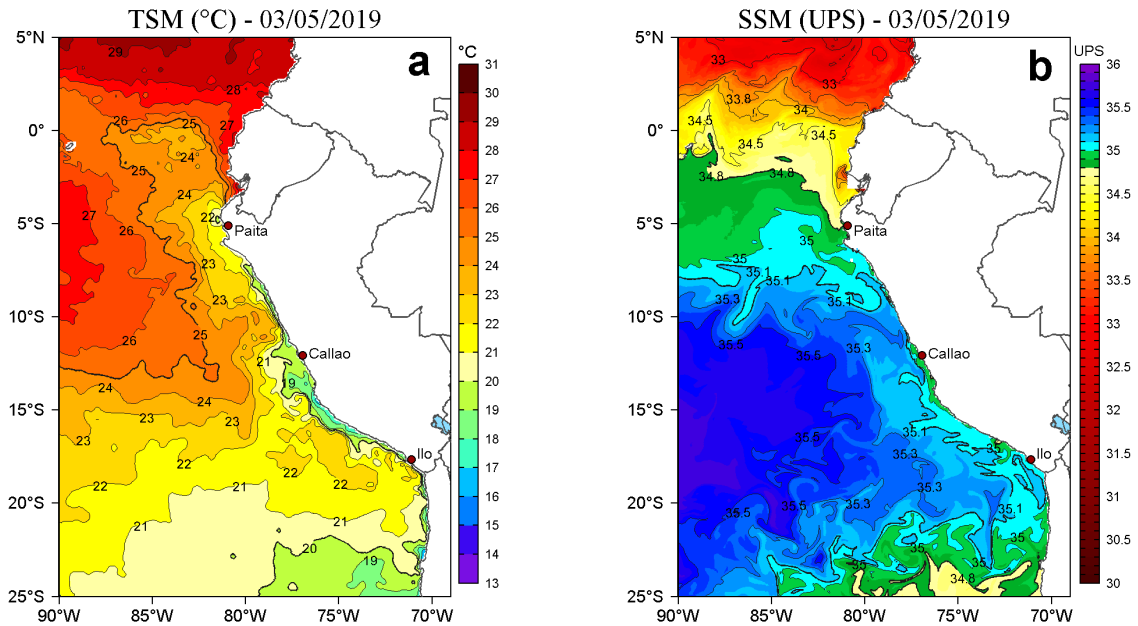
Figura 2. a) Temperatura superficial del mar (TSM, °C) y b) Salinidad superficial del mar (SSM, UPS), para el 03 de mayo de 2019. Datos: OSTIA-UKMO-L4-GLOB-v2.0 (UK Met Office, 2012; Donlon et al, 2012) disponible en https://podaac.jpl.nasa.gov/dataset/OSTIA-UKMO-L4-GLOB-v2.0 para (a) y Hybrid Coordinate Ocean Model v. GOF3 3.1 (HYCOM; Halliwell et al., 1998; 2000; Bleck, 2001) para (b). Procesamiento: LHF/AFIOF/DGIOCC/IMARPE.
