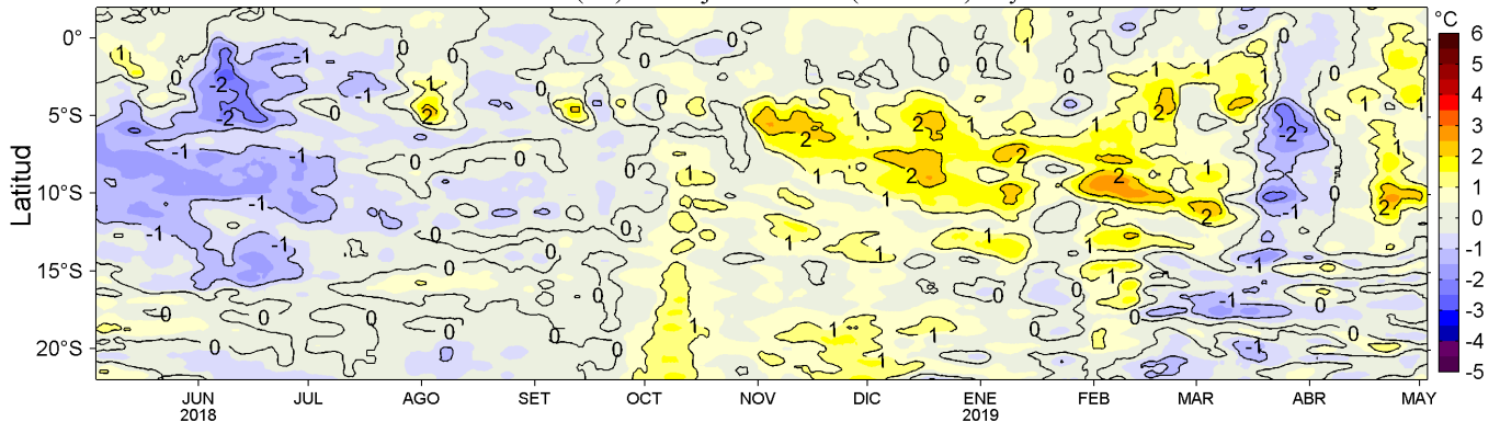
Figura 4. Variación promedio de las anomalías de la temperatura superficial del mar (TSM, °C) para una franja de 60 mn (~111 km) adyacente al litoral peruano para los últimos doce meses al 03 de mayo de 2019. Datos: OSTIA-UKMO-L4-GLOB-v2.0 (UK Met. Office, 2012; Donlon et al, 2012) disponible en https://podaac.jpl.nasa.gov/dataset/OSTIA-UKMO-L4-GLOB-v2.0 . Las anomalías se calcularon con respecto al periodo 2007-2016. Procesamiento: LHF/AFIOF/DGIOCC/IMARPE.
