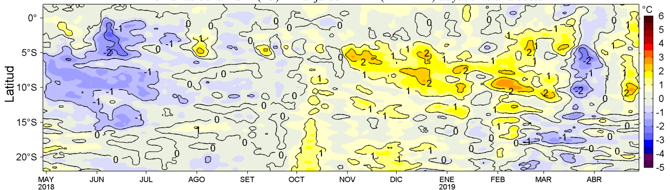
Figura 4. Variación promedio de las anomalías de la temperatura superficial del mar (TSM, °C) para una franja de 60 mn (~111 km) adyacente al litoral peruano para los últimos doce meses al 28 de abril de 2019. Datos: OSTIA-UKMO-L4-GLOB-v2.0 (UK Met. Office, 2012; Donlon et al, 2012) disponible en https://podaac.jpl.nasa.gov/dataset/OSTIA-UKMO-L4-GLOB-v2.0 . Las anomalías se calcularon con respecto al periodo 2007-2016. Procesamiento: LHF/AFIOF/DGIOCC/IMARPE.
