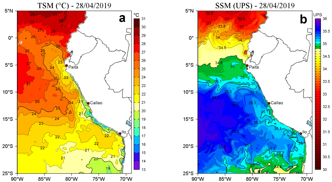
Figura 2. a) Temperatura superficial del mar (TSM, °C) y b) Salinidad superficial del mar (SSM, UPS), para el 28 de abril de 2019. Datos: OSTIA-UKMO-L4-GLOB-v2.0 (UK Met Office, 2012; Donlon et al, 2012) disponible en https://podaac.jpl.nasa.gov/dataset/OSTIA-UKMO-L4-GLOB-v2.0 para (a) y Hybrid Coordinate Ocean Model v. GOF3 3.1 (HYCOM; Halliwell et al., 1998; 2000; Bleck, 2001) para (b). Procesamiento: LHF/AFIOF/DGIOCC/IMARPE.
