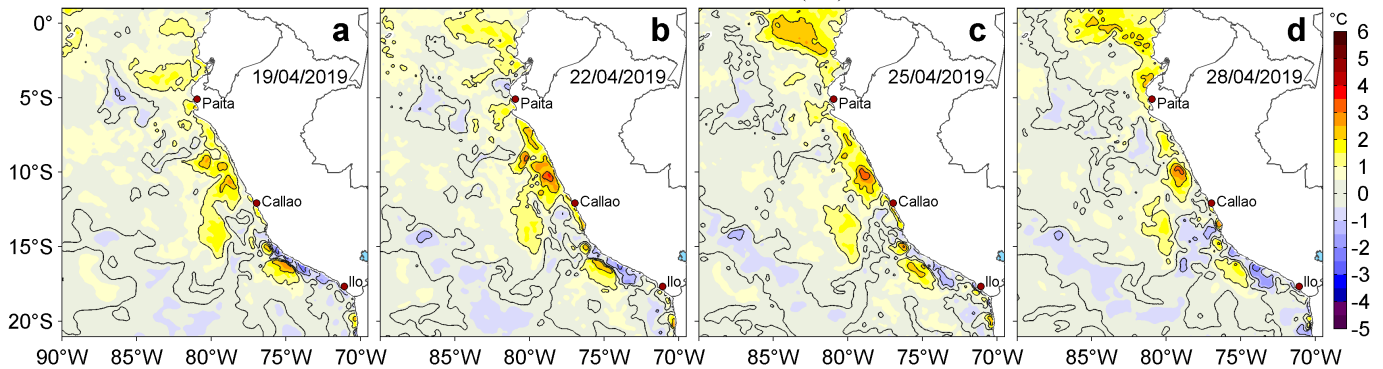
Figura 3. Anomalías de la temperatura superficial del mar (TSM, °C) para los días: a) 19, b) 22, c) 25 y d) 28 de abril de 2019. Las anomalías se calcularon respecto de la climatología para el periodo 2007-2016. Datos: OSTIA-UKMO-L4-GLOB-v2.0 (UK Met Office, 2012; Donlon et al, 2012). Procesamiento: LHF/AFIOF/DGIOCC/IMARPE.
