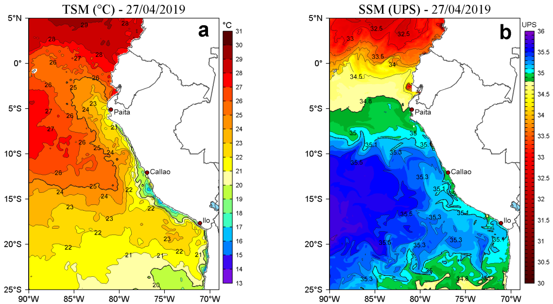
Figura 2. a) Temperatura superficial del mar (TSM, °C) y b) Salinidad superficial del mar (SSM, UPS), para el 27 de abril de 2019. Datos: OSTIA-UKMO-L4-GLOB-v2.0 (UK Met Office, 2012; Donlon et al, 2012) disponible en https://podaac.jpl.nasa.gov/dataset/OSTIA-UKMO-L4-GLOB-v2.0 para (a) y Hybrid Coordinate Ocean Model v. GOF3 3.1 (HYCOM; Halliwell et al., 1998; 2000; Bleck, 2001) para (b). Procesamiento: LHF/AFIOF/DGIOCC/IMARPE.
