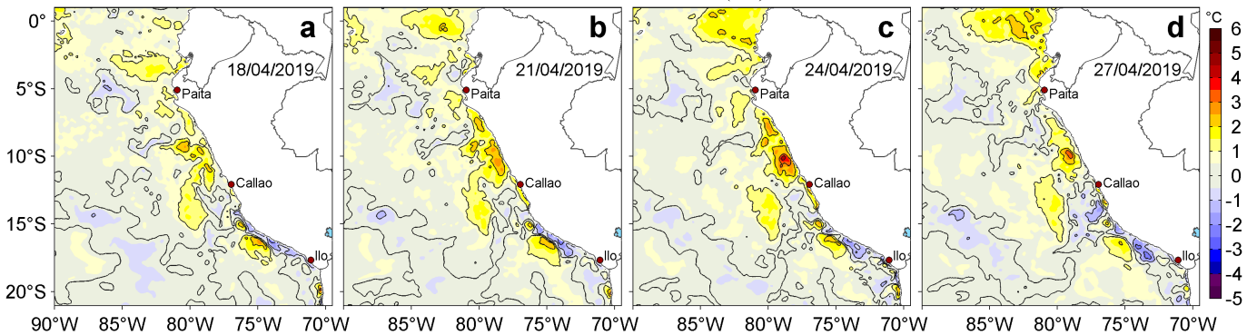
Figura 3. Anomalías de la temperatura superficial del mar (TSM, °C) para los días: a) 18, b) 21, c) 24 y d) 27 de abril de 2019. Las anomalías se calcularon respecto de la climatología para el periodo 2007-2016. Datos: OSTIA-UKMO-L4-GLOB-v2.0 (UK Met Office, 2012; Donlon et al, 2012). Procesamiento: LHF/AFIOF/DGIOCC/IMARPE.
