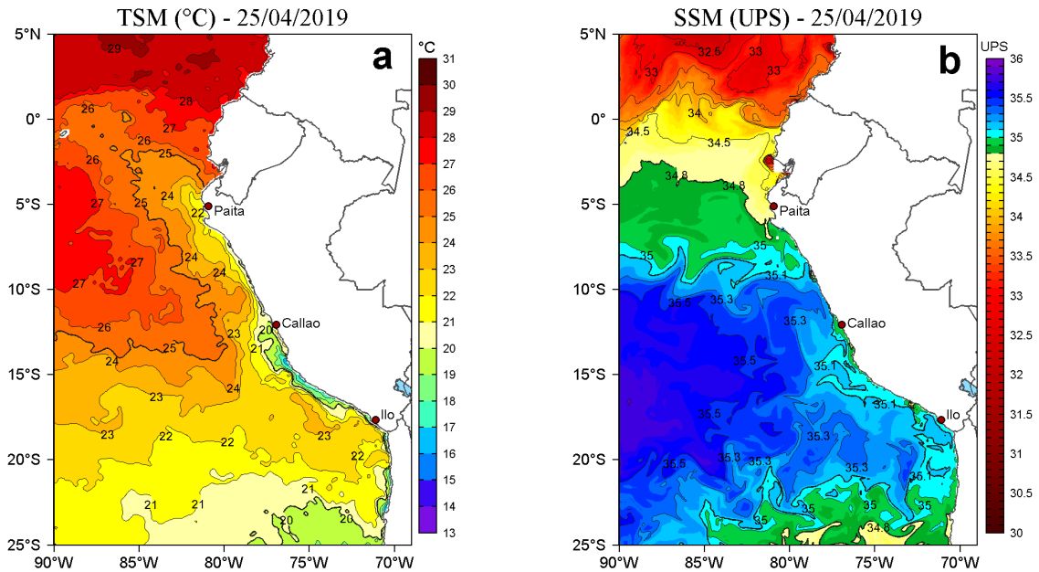
Figura 2. a) Temperatura superficial del mar (TSM, °C) y b) Salinidad superficial del mar (SSM, UPS), para el 25 de abril de 2019. Datos: OSTIA-UKMO-L4-GLOB-v2.0 (UK Met Office, 2012; Donlon et al, 2012) disponible en https://podaac.jpl.nasa.gov/dataset/OSTIA-UKMO-L4-GLOB-v2.0 para (a) y Hybrid Coordinate Ocean Model v. GOF3 3.1 (HYCOM; Halliwell et al., 1998; 2000; Bleck, 2001) para (b). Procesamiento: LHFm/AFIOF/DGIOCC/IMARPE.
