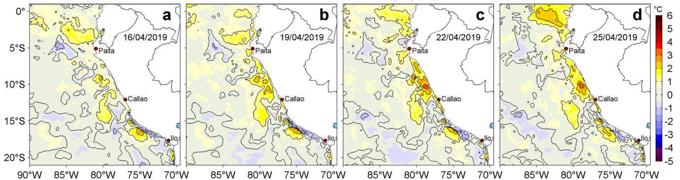
Figura 3. Anomalías de la temperatura superficial del mar (TSM, °C) para los días: a) 16, b) 19, c) 22 y d) 25 de abril de 2019. Las anomalías se calcularon respecto de la climatología para el periodo 2007-2016. Datos: OSTIA-UKMO-L4-GLOB-v2.0 (UK Met Office, 2012; Donlon et al, 2012). Procesamiento: LHFm/AFIOF/DGIOCC/IMARPE.
