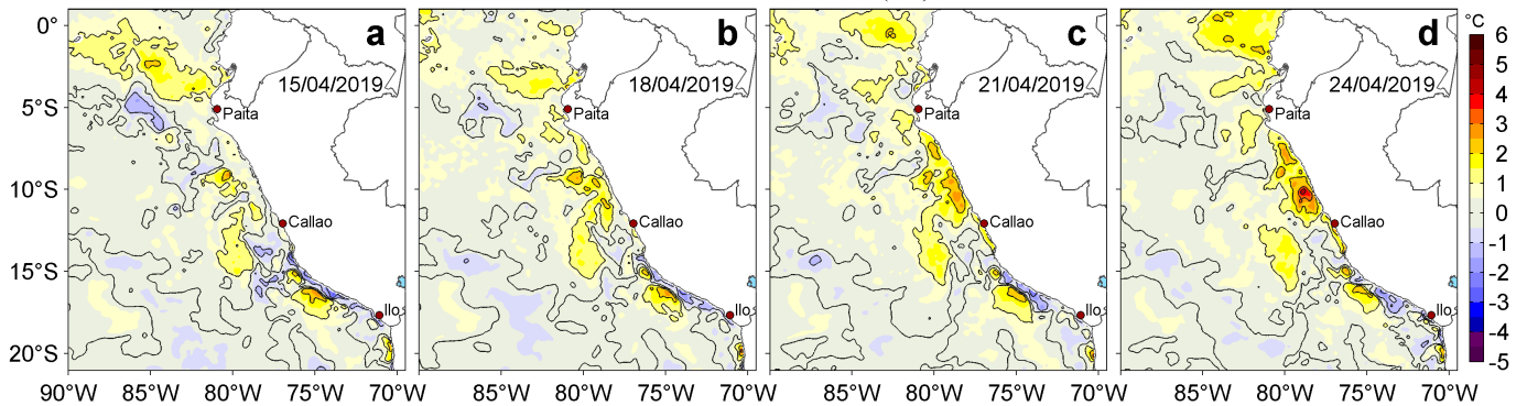
Figura 3. Anomalías de la temperatura superficial del mar (TSM, °C) para los días: a) 15, b) 18, c) 21 y d) 24 de abril de 2019. Las anomalías se calcularon respecto de la climatología para el periodo 2007-2016. Datos: OSTIA-UKMO-L4-GLOB-v2.0 (UK Met Office, 2012; Donlon et al, 2012). Procesamiento: LHF/AFIOF/DGIOCC/IMARPE.
