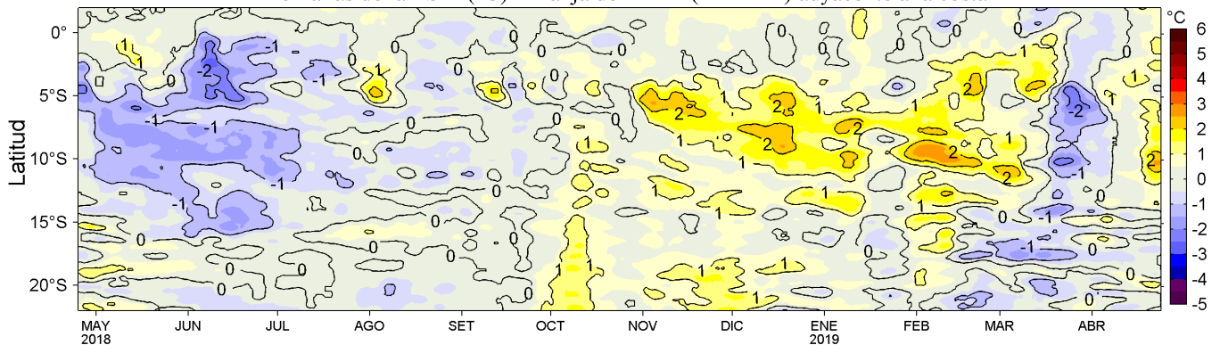
Figura 4. Variación promedio de las anomalías de la temperatura superficial del mar (TSM, °C) para una franja de 60 mn (~111 km) adyacente al litoral peruano para los últimos doce meses al 24 de abril de 2019. Datos: OSTIA-UKMO-L4-GLOB-v2.0 (UK Met. Office, 2012; Donlon et al, 2012) disponible en https://podaac.jpl.nasa.gov/dataset/OSTIA-UKMO-L4-GLOB-v2.0 . Las anomalías se calcularon con respecto al periodo 2007-2016. Procesamiento: LHF/AFIOF/DGIOCC/IMARPE.
