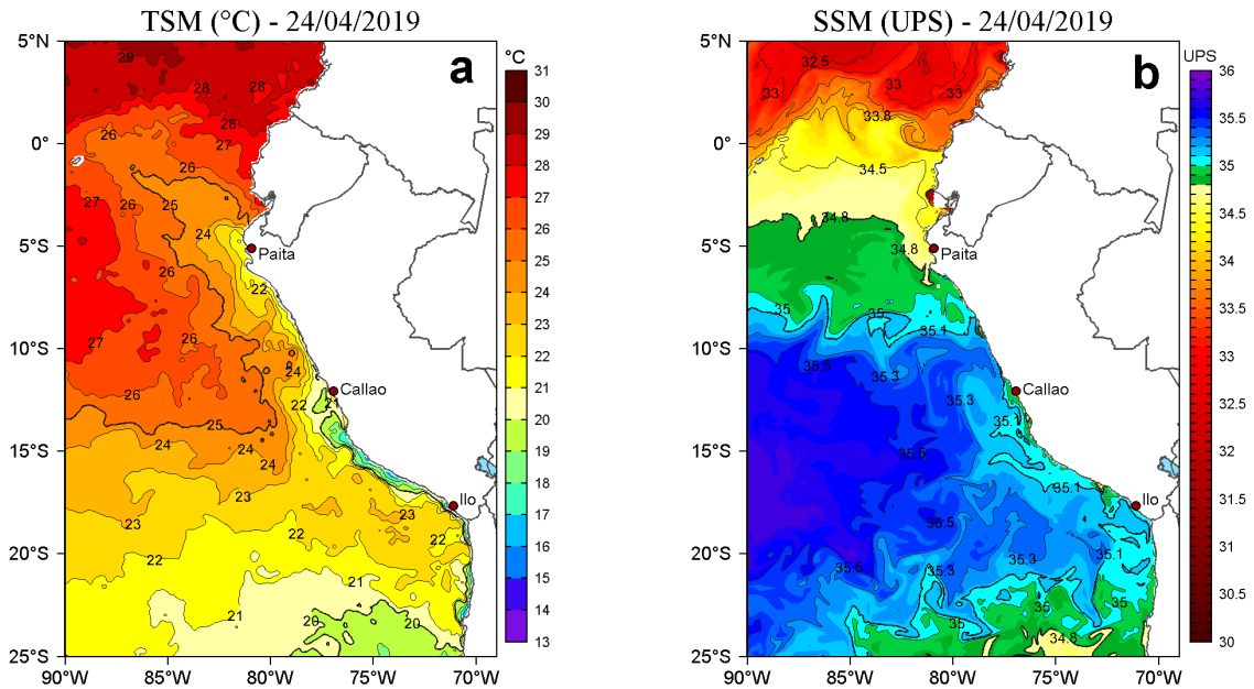
Figura 2. a) Temperatura superficial del mar (TSM, °C) y b) Salinidad superficial del mar (SSM, UPS), para el 24 de abril de 2019. Datos: OSTIA-UKMO-L4-GLOB-v2.0 (UK Met Office, 2012; Donlon et al, 2012) disponible en https://podaac.jpl.nasa.gov/dataset/OSTIA-UKMO-L4-GLOB-v2.0 para (a) y Hybrid Coordinate Ocean Model v. GOF3 3.1 (HYCOM; Halliwell et al., 1998; 2000; Bleck, 2001) para (b). Procesamiento: LHF/AFIOF/DGIOCC/IMARPE.
