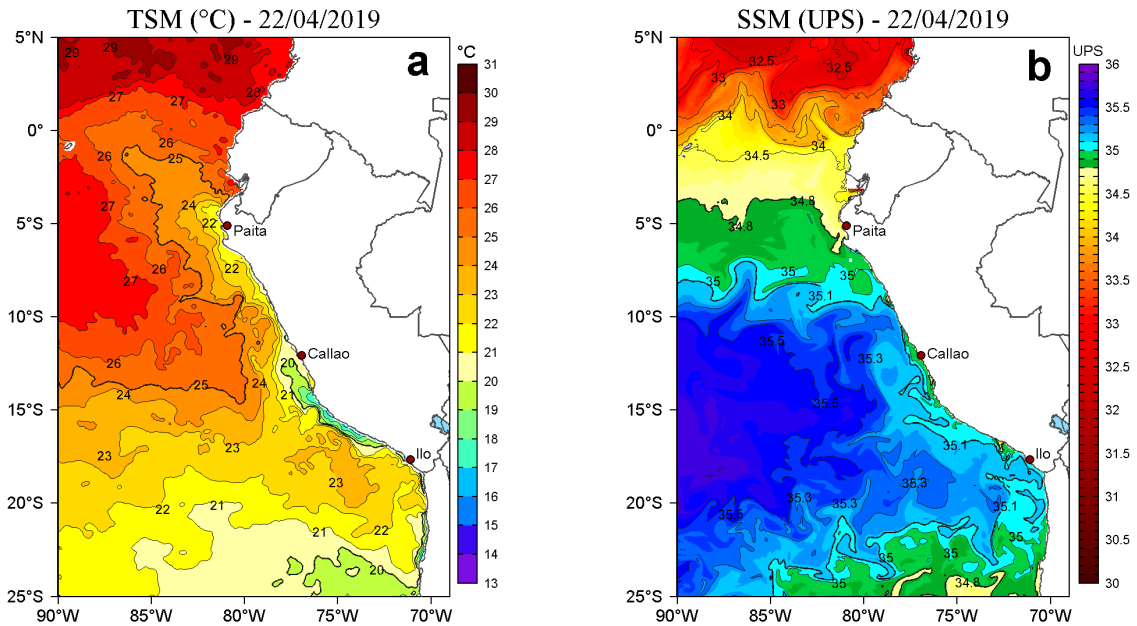
Figura 2. a) Temperatura superficial del mar (TSM, °C) y b) Salinidad superficial del mar (SSM, UPS), para el 22 de abril de 2019. Datos: OSTIA-UKMO-L4-GLOB-v2.0 (UK Met Office, 2012; Donlon et al, 2012) disponible en https://podaac.jpl.nasa.gov/dataset/OSTIA-UKMO-L4-GLOB-v2.0 para (a) y Hybrid Coordinate Ocean Model v. GOF3 3.1 (HYCOM; Halliwell et al., 1998; 2000; Bleck, 2001) para (b). Procesamiento: LHF/AFIOF/DGIOCC/IMARPE.
