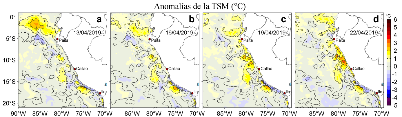
Figura 3. Anomalías de la temperatura superficial del mar (TSM, °C) para los días: a) 13, b) 16, c) 19 y d) 22 de abril de 2019. Las anomalías se calcularon respecto de la climatología para el periodo 2007-2016. Datos: OSTIA-UKMO-L4-GLOB-v2.0 (UK Met Office, 2012; Donlon et al, 2012). Procesamiento: LHF/AFIOF/DGIOCC/IMARPE.
