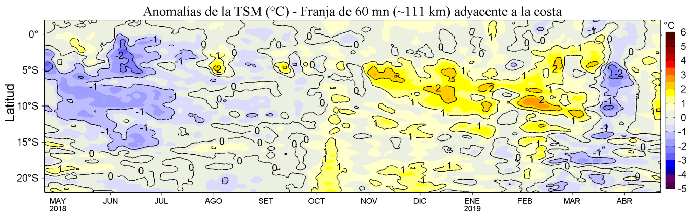
Figura 4. Variación promedio de las anomalías de la temperatura superficial del mar (TSM, °C) para una franja de 60 mn (~111 km) adyacente al litoral peruano para los últimos doce meses al 22 de abril de 2019. Datos: OSTIA-UKMO-L4-GLOB-v2.0 (UK Met. Office, 2012; Donlon et al, 2012) disponible en https://podaac.jpl.nasa.gov/dataset/OSTIA-UKMO-L4-GLOB-v2.0 . Las anomalías se calcularon con respecto al periodo 2007-2016. Procesamiento: LHF/AFIOF/DGIOCC/IMARPE.
