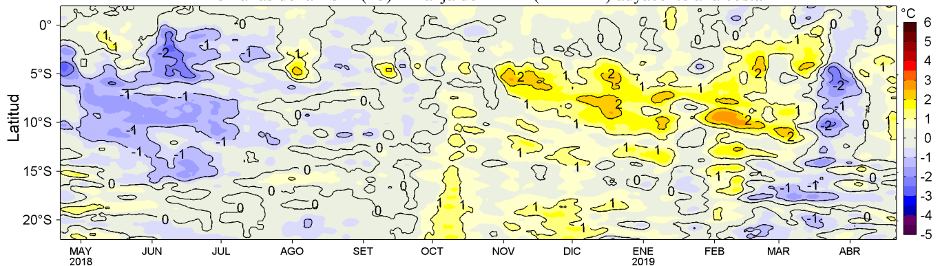
Figura 4. Variación promedio de las anomalías de la temperatura superficial del mar (TSM, °C) para una franja de 60 mn (~111 km) adyacente al litoral peruano para los últimos doce meses al 21 de abril de 2019. Datos: OSTIA-UKMO-L4-GLOB-v2.0 (UK Met. Office, 2012; Donlon et al, 2012) disponible en https://podaac.jpl.nasa.gov/dataset/OSTIA-UKMO-L4-GLOB-v2.0 . Las anomalías se calcularon con respecto al periodo 2007-2016. Procesamiento: LHF/AFIOF/DGIOCC/IMARPE.
