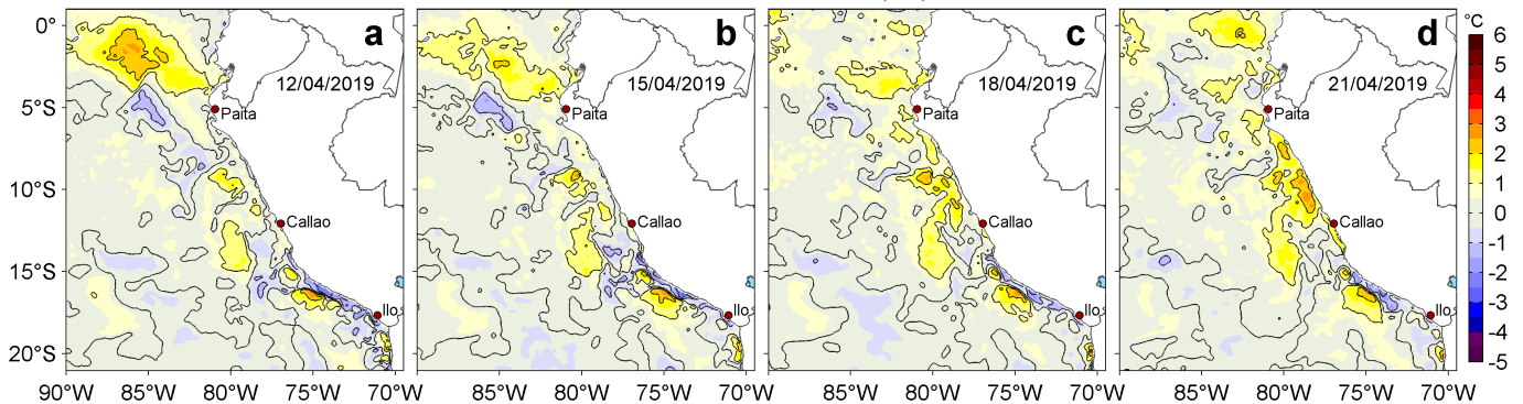
Figura 3. Anomalías de la temperatura superficial del mar (TSM, °C) para los días: a) 12, b) 15, c) 18 y d) 21 de abril de 2019. Las anomalías se calcularon respecto de la climatología para el periodo 2007-2016. Datos: OSTIA-UKMO-L4-GLOB-v2.0 (UK Met Office, 2012; Donlon et al, 2012). Procesamiento: LHF/AFIOF/DGIOCC/IMARPE.
