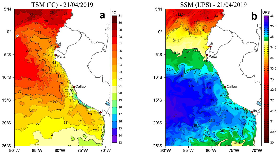
Figura 2. a) Temperatura superficial del mar (TSM, °C) y b) Salinidad superficial del mar (SSM, UPS), para el 21 de abril de 2019. Datos: OSTIA-UKMO-L4-GLOB-v2.0 (UK Met Office, 2012; Donlon et al, 2012) disponible en https://podaac.jpl.nasa.gov/dataset/OSTIA-UKMO-L4-GLOB-v2.0 para (a) y Hybrid Coordinate Ocean Model v. GOF3 3.1 (HYCOM; Halliwell et al., 1998; 2000; Bleck, 2001) para (b). Procesamiento: LHF/AFIOF/DGIOCC/IMARPE.
