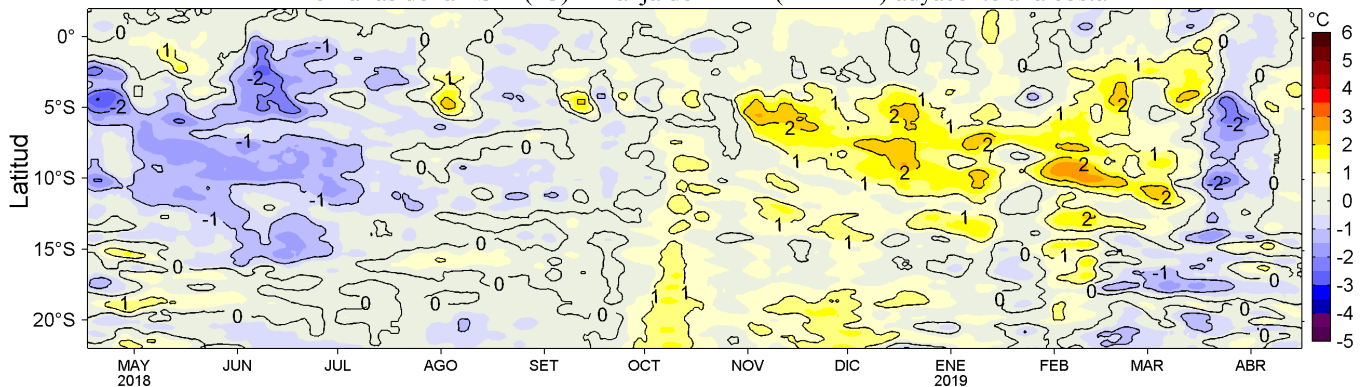
Figura 4. Variación promedio de las anomalías de la temperatura superficial del mar (TSM, °C) para una franja de 60 mn (~111 km) adyacente al litoral peruano para los últimos doce meses al 16 de abril de 2019. Datos: OSTIA-UKMO-L4-GLOB-v2.0 (UK Met. Office, 2012; Donlon et al, 2012) disponible en https://podaac.jpl.nasa.gov/dataset/OSTIA-UKMO-L4-GLOB-v2.0 . Las anomalías se calcularon con respecto al periodo 2007-2016. Procesamiento: LHF/AFIOF/DGIOCC/IMARPE.
