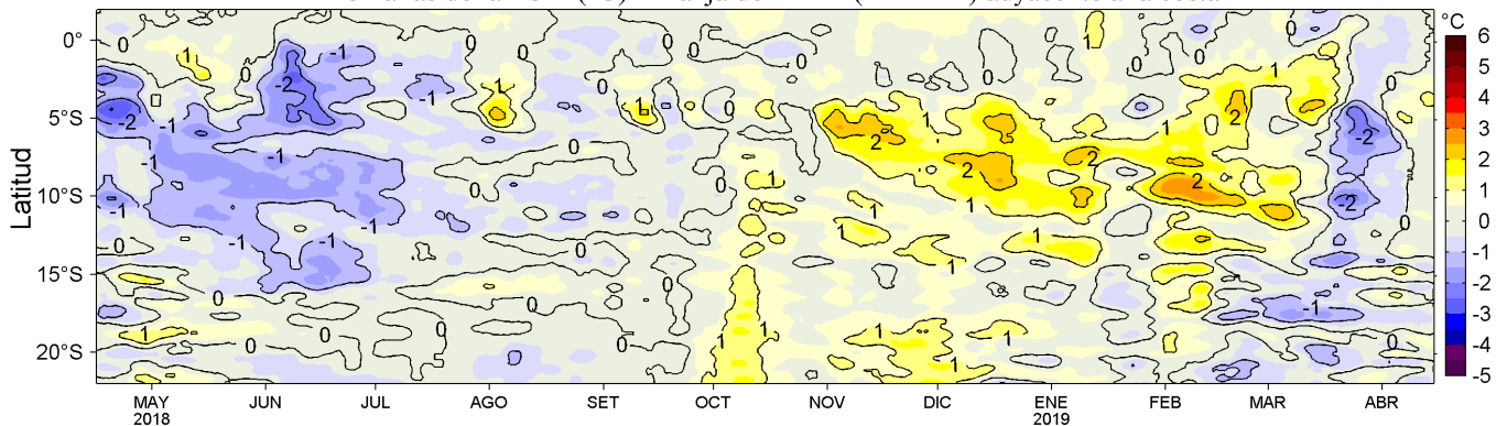
Figura 4. Variación promedio de las anomalías de la temperatura superficial del mar (TSM, °C) para una franja de 60 mn (~111 km) adyacente al litoral peruano para los últimos doce meses al 15 de abril de 2019. Datos: OSTIA-UKMO-L4-GLOB-v2.0 (UK Met. Office, 2012; Donlon et al, 2012) disponible en https://podaac.jpl.nasa.gov/dataset/OSTIA-UKMO-L4-GLOB-v2.0 . Las anomalías se calcularon con respecto al periodo 2007-2016. Procesamiento: LHF/AFIOF/DGIOCC/IMARPE.
