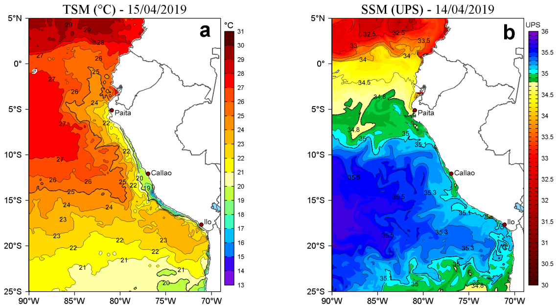
Figura 2. a) Temperatura superficial del mar (TSM, °C) y b) Salinidad superficial del mar (SSM, UPS), para el 15 (TSM) y 14 (SSM) de abril de 2019. Datos: OSTIA-UKMO-L4-GLOB-v2.0 (UK Met Office, 2012; Donlon et al, 2012) disponible en https://podaac.jpl.nasa.gov/dataset/OSTIA-UKMO-L4-GLOB-v2.0 para (a) y Hybrid Coordinate Ocean Model v. GOFS 3.1 (HYCOM; Halliwell et al., 1998; 2000; Bleck, 2001) para (b). Procesamiento: LHF/AFIOF/DGIOCC/IMARPE.
