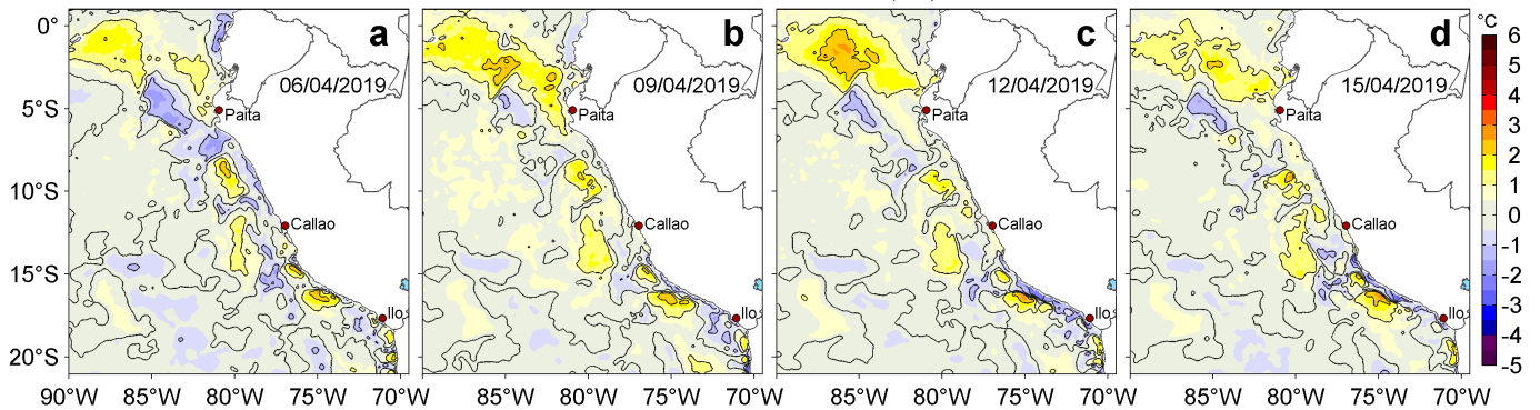
Figura 3. Anomalías de la temperatura superficial del mar (TSM, °C) para los días: a) 06, b) 09, c) 12 y d) 15 de abril de 2019. Las anomalías se calcularon respecto de la climatología para el periodo 2007-2016. Datos: OSTIA-UKMO-L4-GLOB-v2.0 (UK Met Office, 2012; Donlon et al, 2012). Procesamiento: LHF/AFIOF/DGIOCC/IMARPE.
