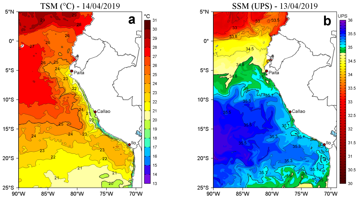
Figura 2. a) Temperatura superficial del mar (TSM, °C) y b) Salinidad superficial del mar (SSM, UPS), para el 14 (TSM) y 13 (SSM) de abril de 2019. Datos: OSTIA-UKMO-L4-GLOB-v2.0 (UK Met Office, 2012; Donlon et al, 2012) disponible en https://podaac.jpl.nasa.gov/dataset/OSTIA-UKMO-L4-GLOB-v2.0 para (a) y Hybrid Coordinate Ocean Model v. GOFS 3.1 (HYCOM; Halliwell et al., 1998; 2000; Bleck, 2001) para (b). Procesamiento: LHF/AFIOF/DGIOCC/IMARPE.
