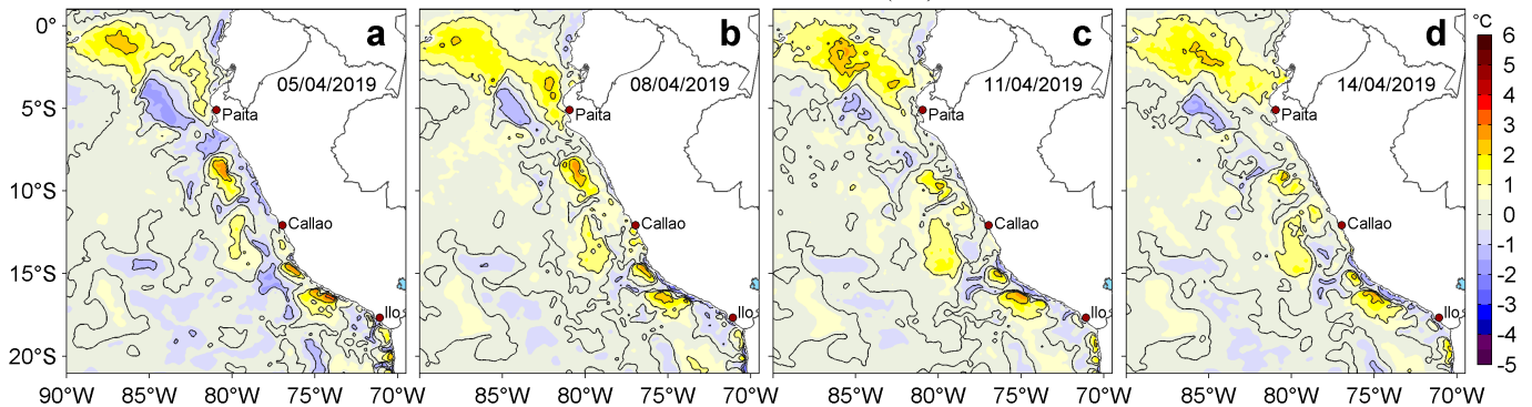
Figura 3. Anomalías de la temperatura superficial del mar (TSM, °C) para los días: a) 05, b) 08, c) 11 y d) 14 de abril de 2019. Las anomalías se calcularon respecto de la climatología para el periodo 2007-2016. Datos: OSTIA-UKMO-L4-GLOB-v2.0 (UK Met Office, 2012; Donlon et al, 2012). Procesamiento: LHF/AFIOF/DGIOCC/IMARPE.
