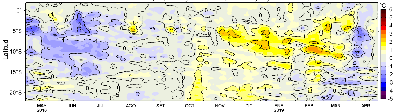
Figura 4. Variación promedio de las anomalías de la temperatura superficial del mar (TSM, °C) para una franja de 60 mn (~111 km) adyacente al litoral peruano para los últimos doce meses al 13 de abril de 2019. Datos: OSTIA-UKMO-L4-GLOB-v2.0 (UK Met. Office, 2012; Donlon et al, 2012) disponible en https://podaac.jpl.nasa.gov/dataset/OSTIA-UKMO-L4-GLOB-v2.0 . Las anomalías se calcularon con respecto al periodo 2007-2016. Procesamiento: LHF/AFIOF/DGIOCC/IMARPE.
