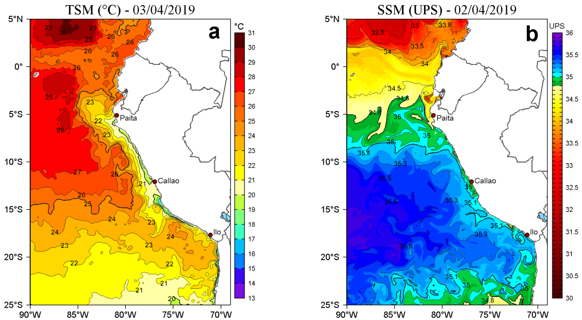
Figura 2. a) Temperatura superficial del mar (TSM, °C) y b) Salinidad superficial del mar (SSM, UPS), para el 03 (TSM) y 02 (SSM) de abril de 2019. Datos: OSTIA-UKMO-L4-GLOB-v2.0 (UK Met Office, 2012; Donlon et al, 2012) disponible en https://podaac.jpl.nasa.gov/dataset/OSTIA-UKMO-L4-GLOB-v2.0 para (a) y Hybrid Coordinate Ocean Model v. GOFS 3.1 (HYCOM; Halliwell et al., 1998; 2000; Bleck, 2001) para (b). Procesamiento: LHF/AFIOF/DGIOCC/IMARPE.
