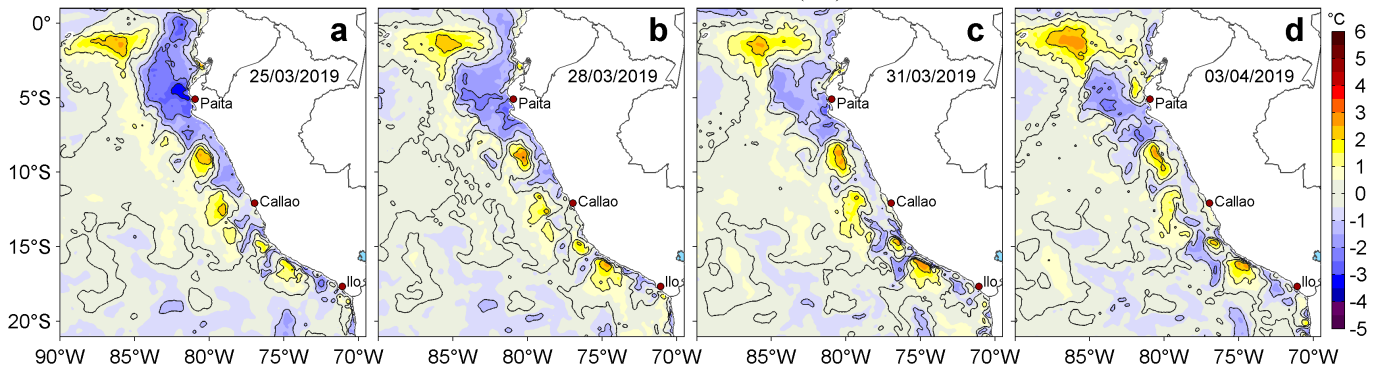
Figura 3. Anomalías de la temperatura superficial del mar (TSM, °C) para los días: a) 25, b) 28 y c) 31 de marzo y d) 03 de abril de 2019. Las anomalías se calcularon respecto de la climatología para el periodo 2007-2016. Datos: OSTIA-UKMO-L4-GLOB-v2.0 (UK Met Office, 2012; Donlon et al, 2012). Procesamiento: LHF/AFIOF/DGIOCC/IMARPE.
