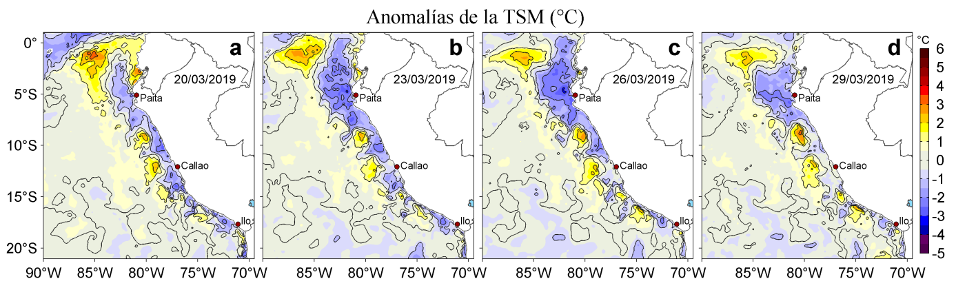
Figura 3. Anomalías de la temperatura superficial del mar (TSM, °C) para los días: a) 20, b) 23, c) 26 y d) 29 de marzo de 2019. Las anomalías se calcularon respecto de la climatología para el periodo 2007-2016. Datos: OSTIA-UKMO-L4-GLOB-v2.0 (UK Met Office, 2012; Donlon et al, 2012). Procesamiento: LHF/AFIOF/DGIOCC/IMARPE.
