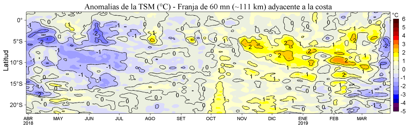
Figura 4. Variación promedio de las anomalías de la temperatura superficial del mar (TSM, °C) para una franja de 60 mn (~111 km) adyacente al litoral peruano para los últimos doce meses al 29 de marzo de 2019. Datos: OSTIA-UKMO-L4-GLOB-v2.0 (UK Met. Office, 2012; Donlon et al, 2012) disponible en https://podaac.jpl.nasa.gov/dataset/OSTIA-UKMO-L4-GLOB-v2.0 . Las anomalías se calcularon con respecto al periodo 2007-2016. Procesamiento: LHF/AFIOF/DGIOCC/IMARPE.
