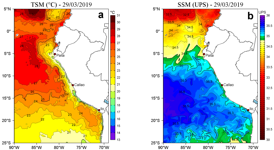
Figura 2. a) Temperatura superficial del mar (TSM, °C) y b) Salinidad superficial del mar (SSM, UPS) para el 29 marzo de 2019. Datos: OSTIA-UKMO-L4-GLOB-v2.0 (UK Met Office, 2012; Donlon et al, 2012) disponible en https://podaac.jpl.nasa.gov/dataset/OSTIA-UKMO-L4-GLOB-v2.0 para (a) y Hybrid Coordinate Ocean Model v. GOF3.1 (HYCOM; Halliwell et al., 1998; 2000; Bleck, 2001) para (b). Procesamiento: LHF/AFIOF/DGIOCC/IMARPE.
