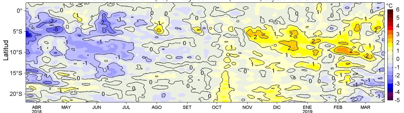
Figura 4. Variación promedio de las anomalías de la temperatura superficial del mar (TSM, °C) para una franja de 60 mn (~111 km) adyacente al litoral peruano para los últimos doce meses al 20 de marzo de 2019. Datos: OSTIA-UKMO-L4-GLOB-v2.0 (UK Met. Office, 2012; Donlon et al, 2012) disponible en https://podaac.jpl.nasa.gov/dataset/OSTIA-UKMO-L4-GLOB-v2.0 . Las anomalías se calcularon con respecto al periodo 2007-2016. Procesamiento: LHF/AFIOF/DGIOCC/IMARPE.
