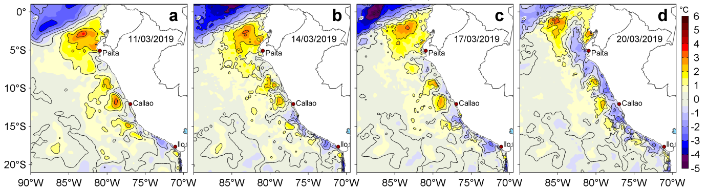
Figura 3. Anomalías de la temperatura superficial del mar (TSM, °C) para los días: a) 11, b) 14, c) 17 y d) 20 de marzo de 2019. Las anomalías se calcularon respecto de la climatología para el periodo 2007-2016. Datos: OSTIA-UKMO-L4-GLOB-v2.0 (UK Met Office, 2012; Donlon et al, 2012). Procesamiento: LHF/AFIOF/DGIOCC/IMARPE.
