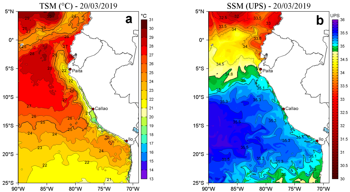
Figura 2. a) Temperatura superficial del mar (TSM, °C) y b) Salinidad superficial del mar (SSM, UPS) para el 20 de marzo de 2019. Datos: OSTIA-UKMO-L4-GLOB-v2.0 (UK Met Office, 2012; Donlon et al, 2012) disponible en https://podaac.jpl.nasa.gov/dataset/OSTIA-UKMO-L4-GLOB-v2.0 para (a) y Hybrid Coordinate Ocean Model v. GOF3.1 (HYCOM; Halliwell et al., 1998; 2000; Bleck, 2001) para (b). Procesamiento: LHF/AFIOF/DGIOCC/IMARPE.
