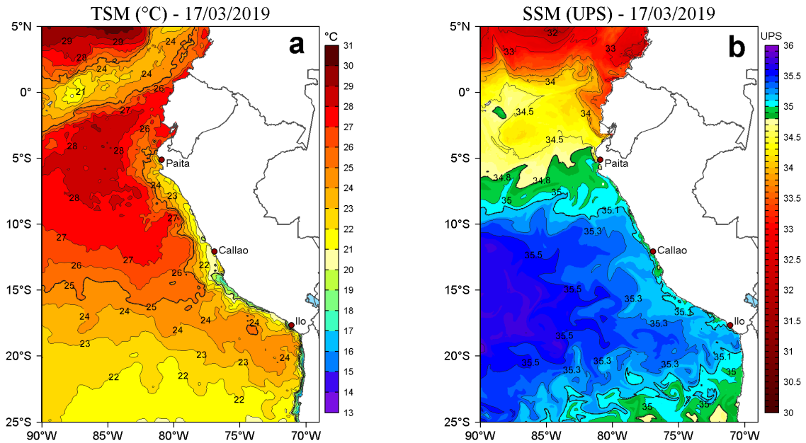
Figura 2. a) Temperatura superficial del mar (TSM, °C) y b) Salinidad superficial del mar (SSM, UPS) para el 17 de marzo de 2019. Datos: OSTIA-UKMO-L4-GLOB-v2.0 (UK Met Office, 2012; Donlon et al, 2012) disponible en https://podaac.jpl.nasa.gov/dataset/OSTIA-UKMO-L4-GLOB-v2.0 para (a) y Hybrid Coordinate Ocean Model v. GOFS 3.1 (HYCOM; Halliwell et al., 1998; 2000; Bleck, 2001) para (b). Procesamiento: LHF/AFIOF/DGIOCC/IMARPE.
