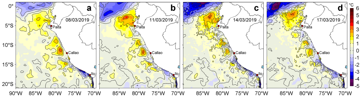
Figura 3. Anomalías de la temperatura superficial del mar (TSM, °C) para los días: a) 08, b) 11, c) 14 y d) 17 de marzo de 2019. Las anomalías se calcularon respecto de la climatología para el periodo 2007-2016. Datos: OSTIA-UKMO-L4-GLOB-v2.0 (UK Met Office, 2012; Donlon et al, 2012). Procesamiento: LHF/AFIOF/DGIOCC/IMARPE.
