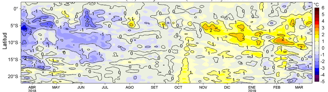
Figura 4. Variación promedio de las anomalías de la temperatura superficial del mar (TSM, °C) para una franja de 60 mn (~111 km) adyacente al litoral peruano para los últimos doce meses al 17 de marzo de 2019. Datos: OSTIA-UKMO-L4-GLOB-v2.0 (UK Met. Office, 2012; Donlon et al, 2012) disponible en https://podaac.jpl.nasa.gov/dataset/OSTIA-UKMO-L4-GLOB-v2.0 . Las anomalías se calcularon con respecto al periodo 2007-2016. Procesamiento: LHF/AFIOF/DGIOCC/IMARPE.
