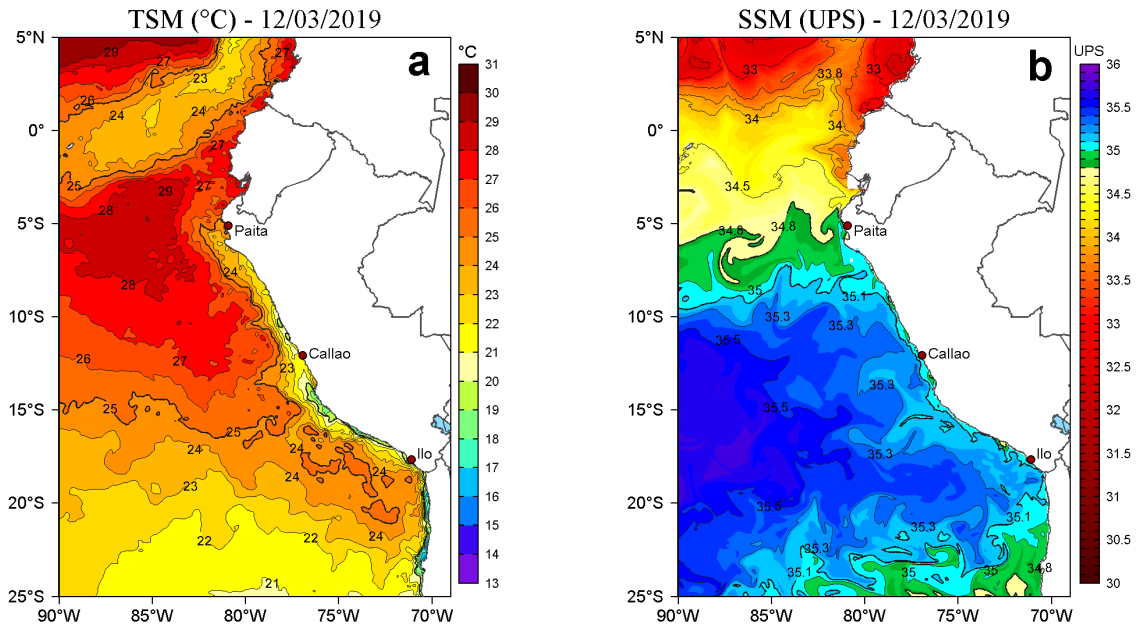
Figura 2. a) Temperatura superficial del mar (TSM, °C) y b) Salinidad superficial del mar (SSM, UPS) para el 12 de marzo de 2019. Datos: OSTIA-UKMO-L4-GLOB-v2.0 (UK Met Office, 2012; Donlon et al, 2012) disponible en https://podaac.jpl.nasa.gov/dataset/OSTIA-UKMO-L4-GLOB-v2.0 para (a) y Hybrid Coordinate Ocean Model v. GOFS 3.1 (HYCOM; Halliwell et al., 1998; 2000; Bleck, 2001) para (b). Procesamiento: LHF/AFIOF/DGIOCC/IMARPE.
