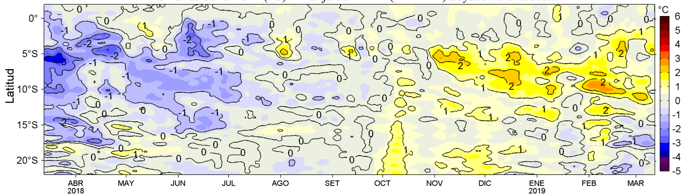
Figura 4. Variación promedio de las anomalías de la temperatura superficial del mar (TSM, °C) para una franja de 60 mn (~111 km) adyacente al litoral peruano para los últimos doce meses al 12 de marzo de 2019. Datos: OSTIA-UKMO-L4-GLOB-v2.0 (UK Met. Office, 2012; Donlon et al, 2012) disponible en https://podaac.jpl.nasa.gov/dataset/OSTIA-UKMO-L4-GLOB-v2.0 . Las anomalías se calcularon con respecto al periodo 2007-2016. Procesamiento: LHF/AFIOF/DGIOCC/IMARPE.
