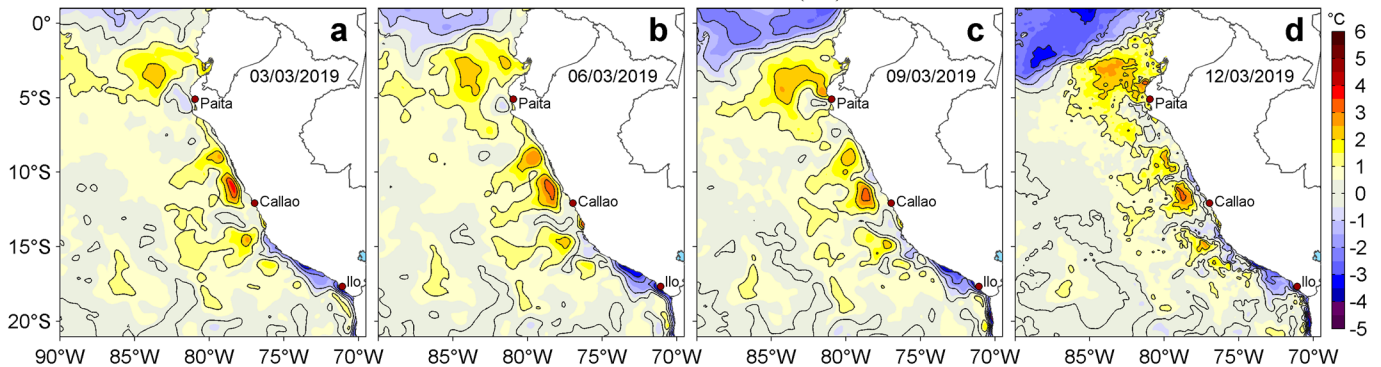
Figura 3. Anomalías de la temperatura superficial del mar (TSM, °C) para los días: a) 03, b) 06, c) 09 y d) 12 de marzo de 2019. Las anomalías se calcularon respecto de la climatología para el periodo 2007-2016. Datos: OSTIA-UKMO-L4-GLOB-v2.0 (UK Met Office, 2012; Donlon et al, 2012). Procesamiento: LHF/AFIOF/DGIOCC/IMARPE.
