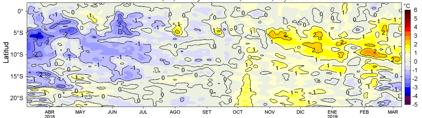
Figura 4. Variación promedio de las anomalías de la temperatura superficial del mar (TSM, °C) para una franja de 60 mn (~111 km) adyacente al litoral peruano para los últimos doce meses al 09 de marzo de 2019. Datos: OSTIA-UKMO-L4-GLOB-v2.0 (UK Met. Office, 2012; Donlon et al, 2012) disponible en https://podaac.jpl.nasa.gov/dataset/OSTIA-UKMO-L4-GLOB-v2.0 . Las anomalías se calcularon con respecto al periodo 2007-2016. Procesamiento: LHFH/AFIOF/DGIOCC/IMARPE.
