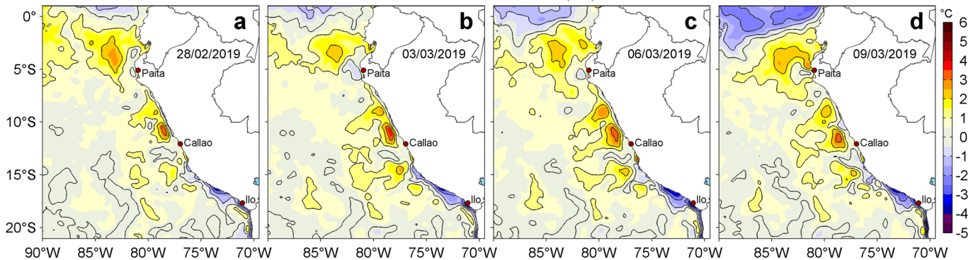
Figura 3. Anomalías de la temperatura superficial del mar (TSM, °C) para los días: a) 28 de febrero, b) 03, c) 06 y d) 09 de marzo de 2019. Las anomalías se calcularon respecto de la climatología para el periodo 2007-2016. Datos: OSTIA-UKMO-L4-GLOB-v2.0 (UK Met Office, 2012; Donlon et al, 2012). Procesamiento: LHFH/AFIOF/DGIOCC/IMARPE.
