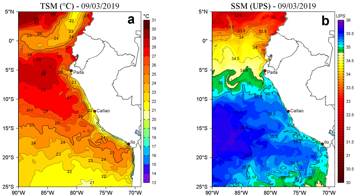
Figura 2. a) Temperatura superficial del mar (TSM, °C) y b) Salinidad superficial del mar (SSM, UPS) para el 09 de marzo de 2019. Datos: OSTIA-UKMO-L4-GLOB-v2.0 (UK Met Office, 2012; Donlon et al, 2012) disponible en https://podaac.jpl.nasa.gov/dataset/OSTIA-UKMO-L4-GLOB-v2.0 para (a) y Hybrid Coordinate Ocean Model v. GOFS 3.1 (HYCOM; Halliwell et al., 1998; 2000; Bleck, 2001) para (b). Procesamiento: LHFH/AFIOF/DGIOCC/IMARPE.
