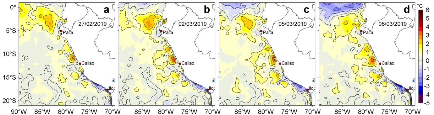
Figura 3. Anomalías de la temperatura superficial del mar (TSM, °C) para los días: a) 27 de febrero, b) 02, c) 05 y d) 08 de marzo de 2019. Las anomalías se calcularon respecto de la climatología para el periodo 2007-2016. Datos: OSTIA-UKMO-L4-GLOB-v2.0 (UK Met Office, 2012; Donlon et al, 2012). Procesamiento: LHFm/AFIOF/DGIOCC/IMARPE.
