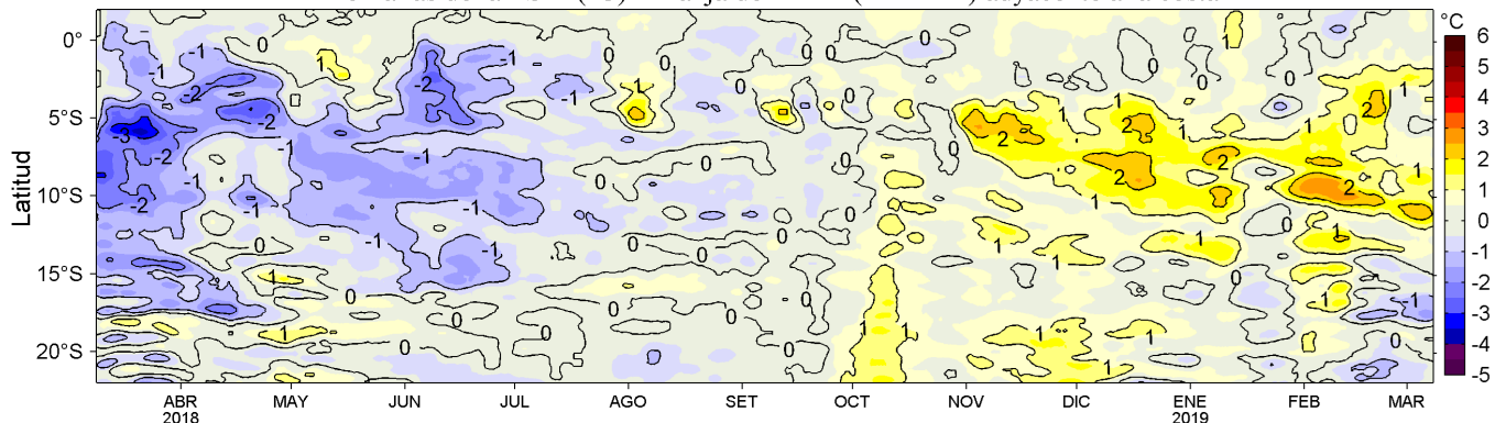
Figura 4. Variación promedio de las anomalías de la temperatura superficial del mar (TSM, °C) para una franja de 60 mn (~111 km) adyacente al litoral peruano para los últimos doce meses al 08 de marzo de 2019. Datos: OSTIA-UKMO-L4-GLOB-v2.0 (UK Met. Office, 2012; Donlon et al, 2012) disponible en https://podaac.jpl.nasa.gov/dataset/OSTIA-UKMO-L4-GLOB-v2.0 . Las anomalías se calcularon con respecto al periodo 2007-2016. Procesamiento: LHFm/AFIOF/DGIOCC/IMARPE.
