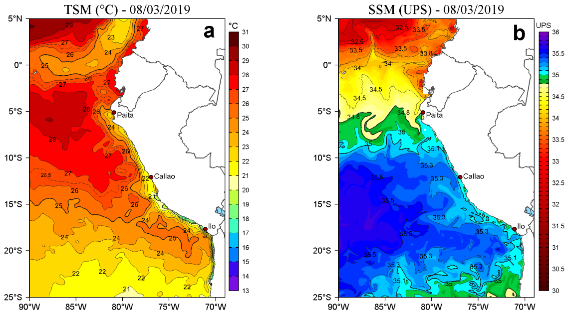
Figura 2. a) Temperatura superficial del mar (TSM, °C) y b) Salinidad superficial del mar (SSM, UPS) para el 08 de marzo de 2019. Datos: OSTIA-UKMO-L4-GLOB-v2.0 (UK Met Office, 2012; Donlon et al, 2012) disponible en https://podaac.jpl.nasa.gov/dataset/OSTIA-UKMO-L4-GLOB-v2.0 para (a) y Hybrid Coordinate Ocean Model v. GOFS 3.1 (HYCOM; Halliwell et al., 1998; 2000; Bleck, 2001) para (b). Procesamiento: LHFm/AFIOF/DGIOCC/IMARPE.
