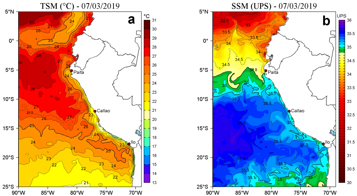
Figura 2. a) Temperatura superficial del mar (TSM, °C) y b) Salinidad superficial del mar (SSM, UPS) para el 07 de marzo de 2019. Datos: OSTIA-UKMO-L4-GLOB-v2.0 (UK Met Office, 2012; Donlon et al, 2012) disponible en https://podaac.jpl.nasa.gov/dataset/OSTIA-UKMO-L4-GLOB-v2.0 para (a) y Hybrid Coordinate Ocean Model v. GOFS 3.1 (HYCOM; Halliwell et al., 1998; 2000; Bleck, 2001) para (b). Procesamiento: LHF/AFIOF/DGIOCC/IMARPE.
