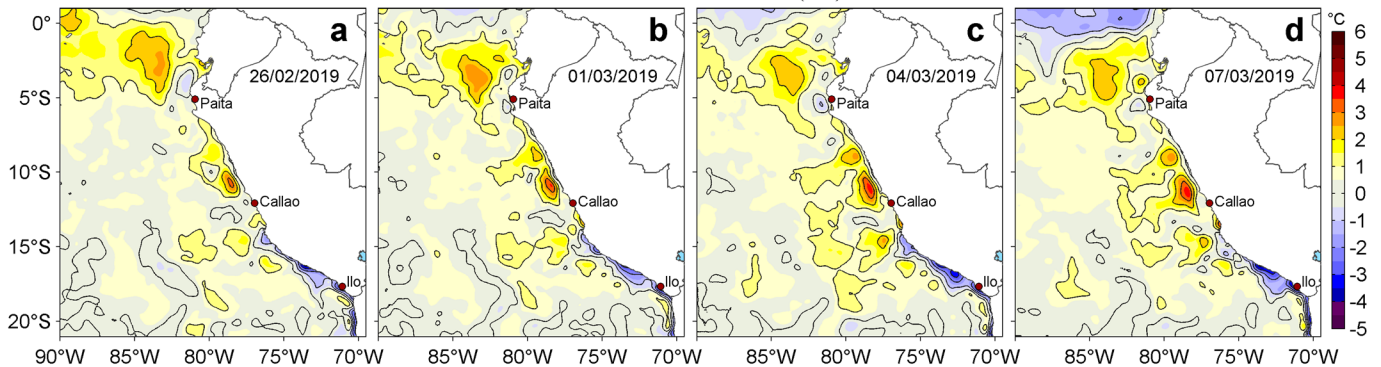
Figura 3. Anomalías de la temperatura superficial del mar (TSM, °C) para los días: a) 26 de febrero, b) 01, c) 04 y d) 07 de marzo de 2019. Las anomalías se calcularon respecto de la climatología para el periodo 2007-2016. Datos: OSTIA-UKMO-L4-GLOB-v2.0 (UK Met Office, 2012; Donlon et al, 2012). Procesamiento: LHF/AFIOF/DGIOCC/IMARPE.
