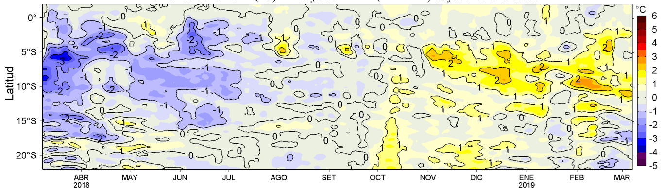
Figura 4. Variación promedio de las anomalías de la temperatura superficial del mar (TSM, °C) para una franja de 60 mn (~111 km) adyacente al litoral peruano para los últimos doce meses al 07 de marzo de 2019. Datos: OSTIA-UKMO-L4-GLOB-v2.0 (UK Met. Office, 2012; Donlon et al, 2012) disponible en https://podaac.jpl.nasa.gov/dataset/OSTIA-UKMO-L4-GLOB-v2.0 . Las anomalías se calcularon con respecto al periodo 2007-2016. Procesamiento: LHF/AFIOF/DGIOCC/IMARPE.
