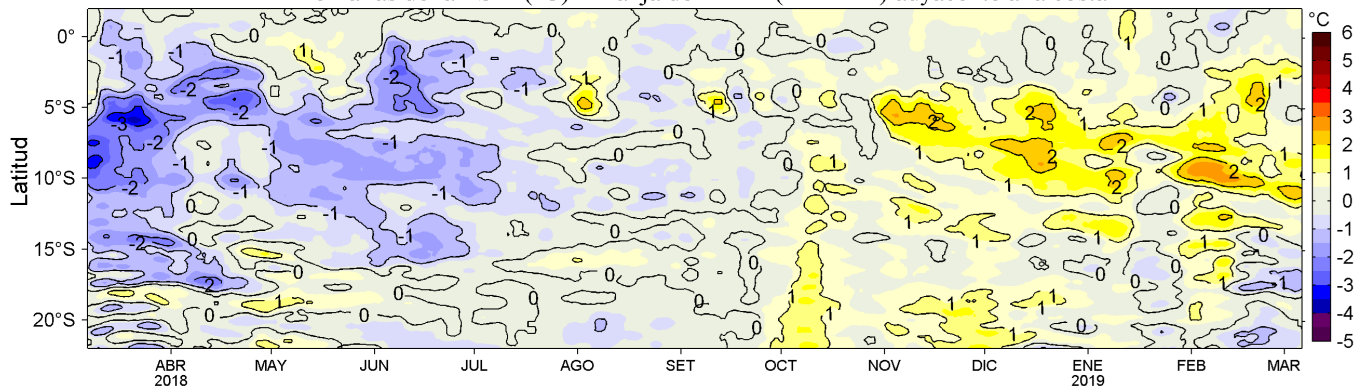
Figura 4. Variación promedio de las anomalías de la temperatura superficial del mar (TSM, °C) para una franja de 60 mn (~111 km) adyacente al litoral peruano para los últimos doce meses al 06 de marzo de 2019. Datos: OSTIA-UKMO-L4-GLOB-v2.0 (UK Met. Office, 2012; Donlon et al, 2012) disponible en https://podaac.jpl.nasa.gov/dataset/OSTIA-UKMO-L4-GLOB-v2.0 . Las anomalías se calcularon con respecto al periodo 2007-2016. Procesamiento: LHF/AFIOF/DGIOCC/IMARPE.
