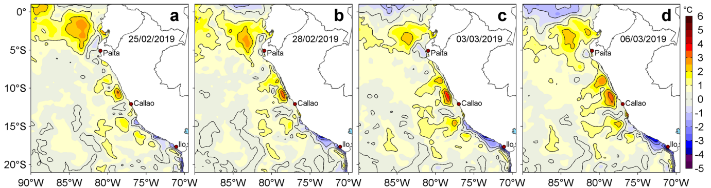
Figura 3. Anomalías de la temperatura superficial del mar (TSM, °C) para los días: a) 25 y b) 28 de febrero, c) 03 y d) 06 de marzo de 2019. Las anomalías se calcularon respecto de la climatología para el periodo 2007-2016. Datos: OSTIA-UKMO-L4-GLOB-v2.0 (UK Met Office, 2012; Donlon et al, 2012). Procesamiento: LHF/AFIOF/DGIOCC/IMARPE.
