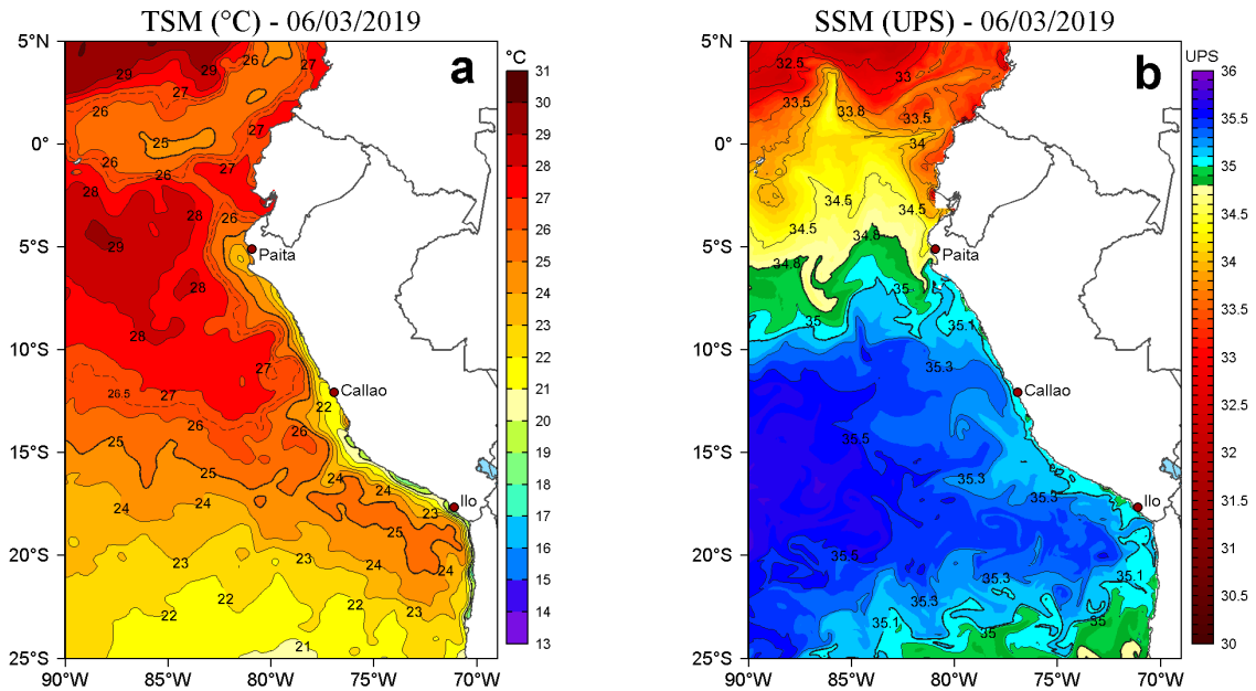
Figura 2. a) Temperatura superficial del mar (TSM, °C) y b) Salinidad superficial del mar (SSM, UPS) para el 06 de marzo de 2019. Datos: OSTIA-UKMO-L4-GLOB-v2.0 (UK Met Office, 2012; Donlon et al, 2012) disponible en https://podaac.jpl.nasa.gov/dataset/OSTIA-UKMO-L4-GLOB-v2.0 para (a) y Hybrid Coordinate Ocean Model v. GOFS 3.1 (HYCOM; Halliwell et al., 1998; 2000; Bleck, 2001) para (b). Procesamiento: LHF/AFIOF/DGIOCC/IMARPE.
