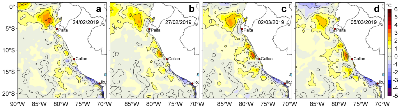
Figura 3. Anomalías de la temperatura superficial del mar (TSM, °C) para los días: a) 24 y b) 27 de febrero, c) 02 y d) 05 de marzo de 2019. Las anomalías se calcularon respecto de la climatología para el periodo 2007-2016. Datos: OSTIA-UKMO-L4-GLOB-v2.0 (UK Met Office, 2012; Donlon et al, 2012). Procesamiento: LHF/AFIOF/DGIOCC/IMARPE.
