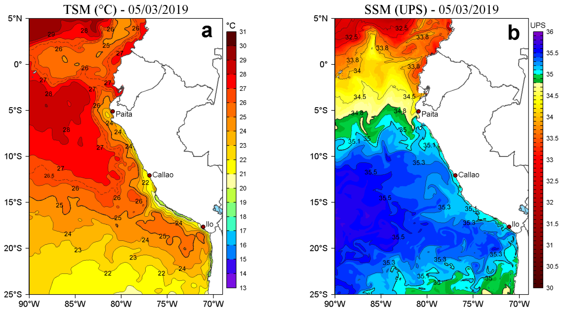
Figura 2. a) Temperatura superficial del mar (TSM, °C) y b) Salinidad superficial del mar (SSM, UPS) para el 05 de marzo de 2019. Datos: OSTIA-UKMO-L4-GLOB-v2.0 (UK Met Office, 2012; Donlon et al, 2012) disponible en https://podaac.jpl.nasa.gov/dataset/OSTIA-UKMO-L4-GLOB-v2.0 para (a) y Hybrid Coordinate Ocean Model v. GOFS 3.1 (HYCOM; Halliwell et al., 1998; 2000; Bleck, 2001) para (b). Procesamiento: LHF/AFIOF/DGIOCC/IMARPE.
