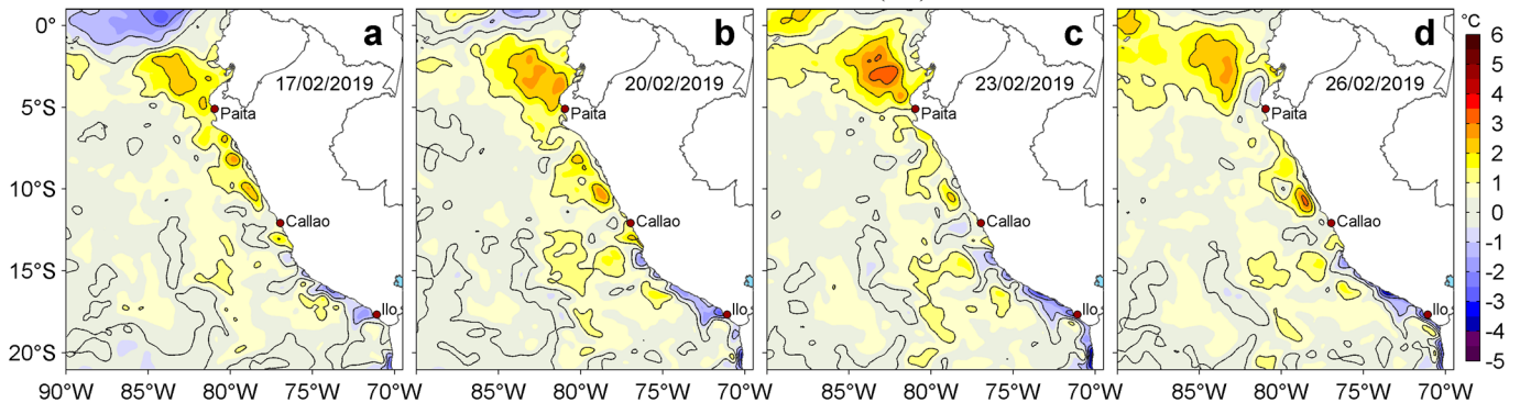
Figura 3. Anomalías de la temperatura superficial del mar (TSM, °C) para los días: a) 17, b) 20, c) 23 y d) 26 de febrero de 2019. Las anomalías se calcularon respecto de la climatología para el periodo 2007-2016. Datos: OSTIA-UKMO-L4-GLOB-v2.0 (UK Met Office, 2012; Donlon et al, 2012). Procesamiento: LHF/AFIOF/DGIOCC/IMARPE.
