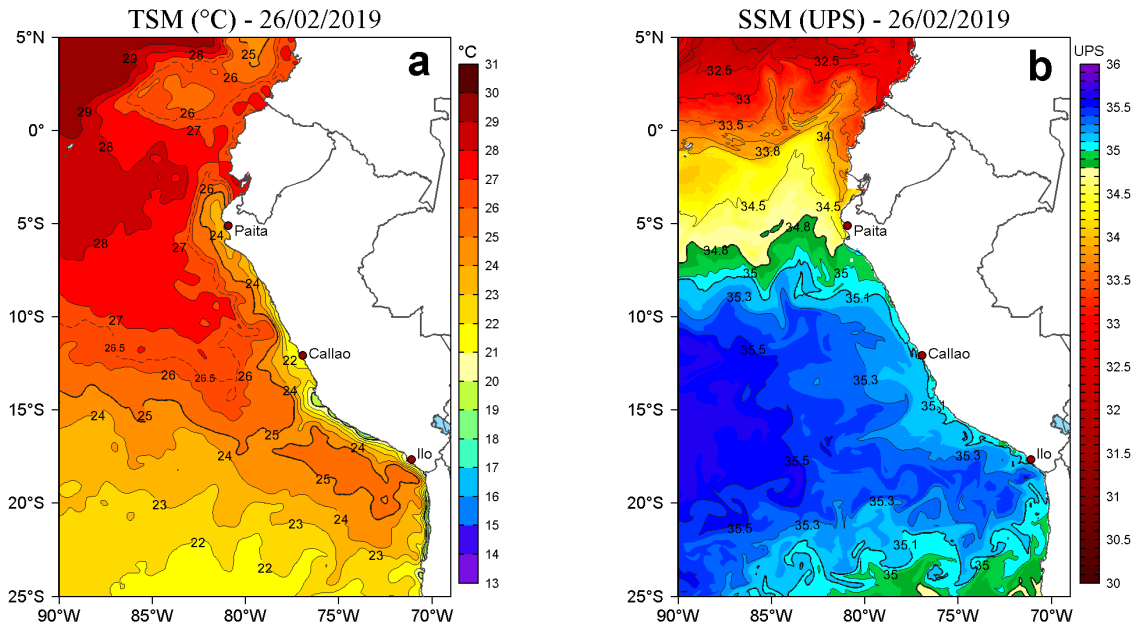
Figura 2. a) Temperatura superficial del mar (TSM, °C) y b) Salinidad superficial del mar (SSM, UPS) para el 26 de febrero de 2019. Datos: OSTIA-UKMO-L4-GLOB-v2.0 (UK Met Office, 2012; Donlon et al, 2012) disponible en https://podaac.jpl.nasa.gov/dataset/OSTIA-UKMO-L4-GLOB-v2.0 para (a) y Hybrid Coordinate Ocean Model v. GOF3 3.1 (HYCOM; Halliwell et al., 1998; 2000; Bleck, 2001) para (b). Procesamiento: LHF/AFIOF/DGIOCC/IMARPE.
