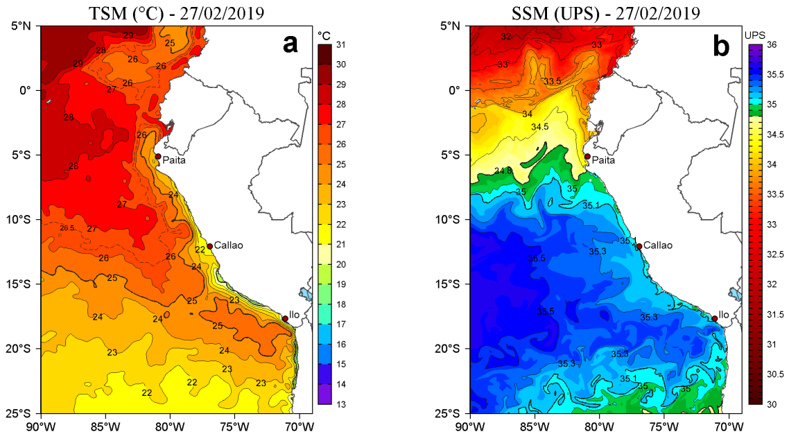
Figura 2. a) Temperatura superficial del mar (TSM, °C) y b) Salinidad superficial del mar (SSM, UPS) para el 27 de febrero de 2019. Datos: OSTIA-UKMO-L4-GLOB-v2.0 (UK Met Office, 2012; Donlon et al, 2012) disponible en https://podaac.jpl.nasa.gov/dataset/OSTIA-UKMO-L4-GLOB-v2.0 para (a) y Hybrid Coordinate Ocean Model v. GOF3 3.1 (HYCOM; Halliwell et al., 1998; 2000; Bleck, 2001) para (b). Procesamiento: LHF/AFIOF/DGIOCC/IMARPE.
