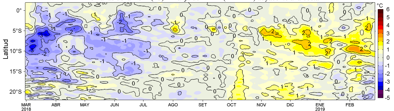
Figura 4. Variación promedio de las anomalías de la temperatura superficial del mar (TSM, °C) para una franja de 60 mn (~111 km) adyacente al litoral peruano para los últimos doce meses al 27 de febrero de 2019. Datos: OSTIA-UKMO-L4-GLOB-v2.0 (UK Met. Office, 2012; Donlon et al, 2012) disponible en https://podaac.jpl.nasa.gov/dataset/OSTIA-UKMO-L4-GLOB-v2.0 . Las anomalías se calcularon con respecto al periodo 2007-2016. Procesamiento: LHF/AFIOF/DGIOCC/IMARPE.
