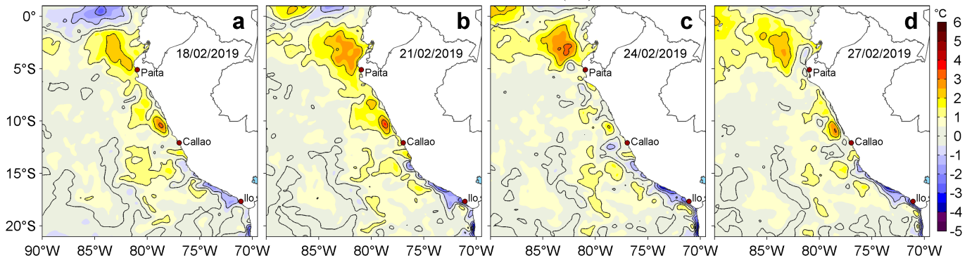
Figura 3. Anomalías de la temperatura superficial del mar (TSM, °C) para los días: a) 18, b) 21, c) 24 y d) 27 de febrero de 2019. Las anomalías se calcularon respecto de la climatología para el periodo 2007-2016. Datos: OSTIA-UKMO-L4-GLOB-v2.0 (UK Met Office, 2012; Donlon et al, 2012). Procesamiento: LHF/AFIOF/DGIOCC/IMARPE.
