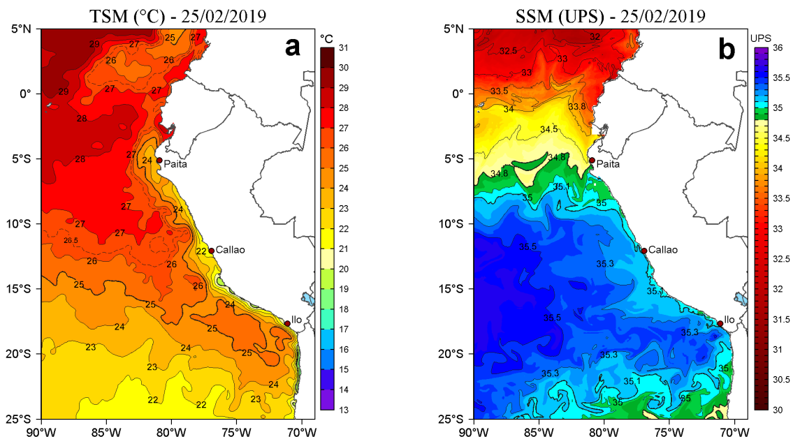
Figura 2. a) Temperatura superficial del mar (TSM, °C) y b) Salinidad superficial del mar (SSM, UPS) para el 25 de febrero de 2019. Datos: OSTIA-UKMO-L4-GLOB-v2.0 (UK Met Office, 2012; Donlon et al, 2012) disponible en https://podaac.jpl.nasa.gov/dataset/OSTIA-UKMO-L4-GLOB-v2.0 para (a) y Hybrid Coordinate Ocean Model v. GOF3 3.1 (HYCOM; Halliwell et al., 1998; 2000; Bleck, 2001) para (b). Procesamiento: LHF/AFIOF/DGIOCC/IMARPE.
