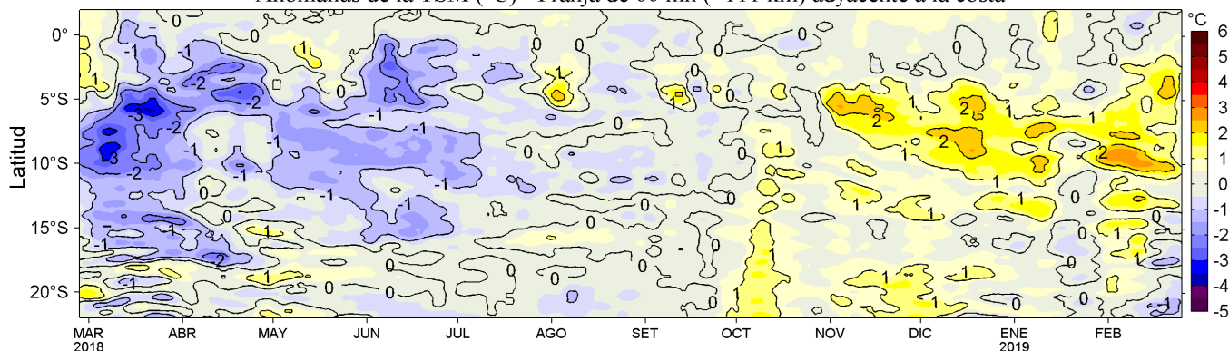
Figura 4. Variación promedio de las anomalías de la temperatura superficial del mar (TSM, °C) para una franja de 60 mn (~111 km) adyacente al litoral peruano para los últimos doce meses al 25 de febrero de 2019. Datos: OSTIA-UKMO-L4-GLOB-v2.0 (UK Met. Office, 2012; Donlon et al, 2012) disponible en https://podaac.jpl.nasa.gov/dataset/OSTIA-UKMO-L4-GLOB-v2.0 . Las anomalías se calcularon con respecto al periodo 2007-2016. Procesamiento: LHF/AFIOF/DGIOCC/IMARPE.
