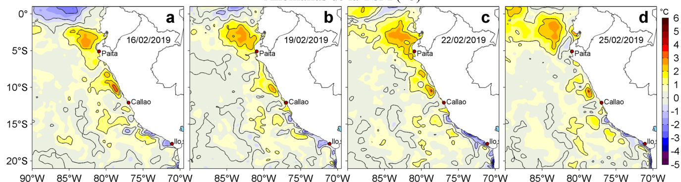
Figura 3. Anomalías de la temperatura superficial del mar (TSM, °C) para los días: a) 16, b) 19, c) 22 y d) 25 de febrero de 2019. Las anomalías se calcularon respecto de la climatología para el periodo 2007-2016. Datos: OSTIA-UKMO-L4-GLOB-v2.0 (UK Met Office, 2012; Donlon et al, 2012). Procesamiento: LHF/AFIOF/DGIOCC/IMARPE.
