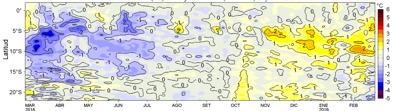
Figura 4. Variación promedio de las anomalías de la temperatura superficial del mar (TSM, °C) para una franja de 60 mn (~111 km) adyacente al litoral peruano para los últimos doce meses al 23 de febrero de 2019. Datos: OSTIA-UKMO-L4-GLOB-v2.0 (UK Met. Office, 2012; Donlon et al, 2012) disponible en https://podaac.jpl.nasa.gov/dataset/OSTIA-UKMO-L4-GLOB-v2.0 . Las anomalías se calcularon con respecto al periodo 2007-2016. Procesamiento: LHF/AFIOF/DGIOCC/IMARPE.
