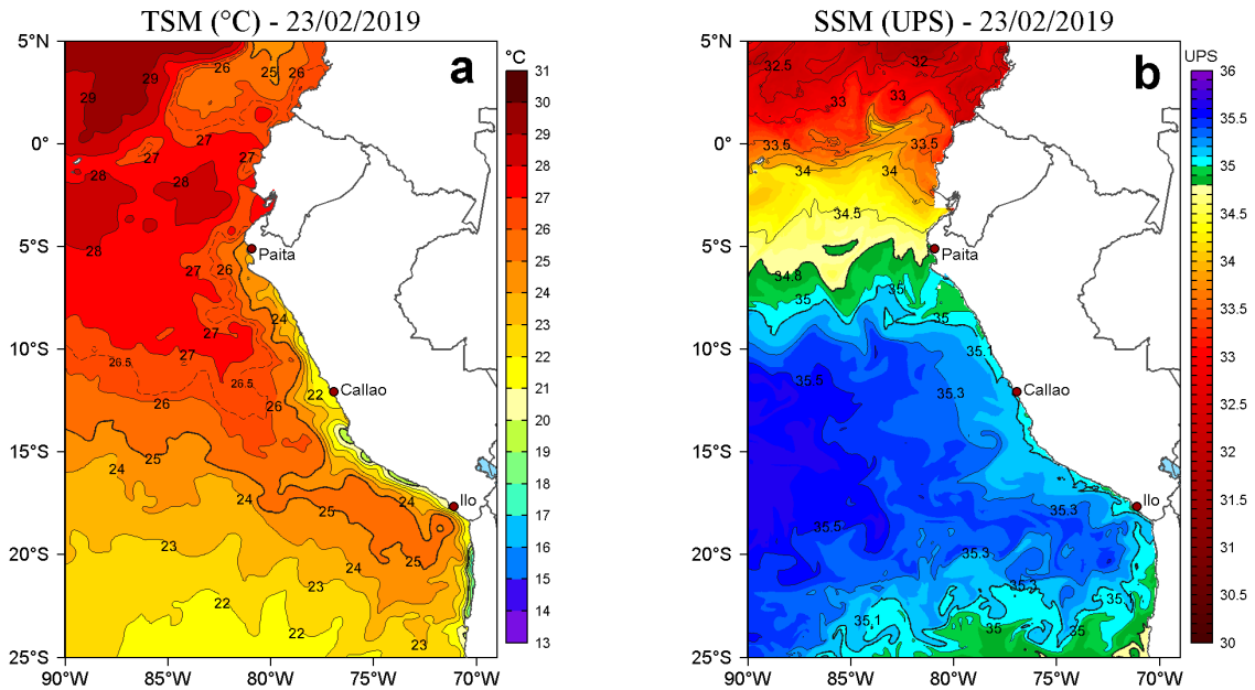
Figura 2. a) Temperatura superficial del mar (TSM, °C) y b) Salinidad superficial del mar (SSM, UPS) para el 23 de febrero de 2019. Datos: OSTIA-UKMO-L4-GLOB-v2.0 (UK Met Office, 2012; Donlon et al, 2012) disponible en https://podaac.jpl.nasa.gov/dataset/OSTIA-UKMO-L4-GLOB-v2.0 para (a) y Hybrid Coordinate Ocean Model v. GOF3 3.1 (HYCOM; Halliwell et al., 1998; 2000; Bleck, 2001) para (b). Procesamiento: LHF/AFIOF/DGIOCC/IMARPE.
