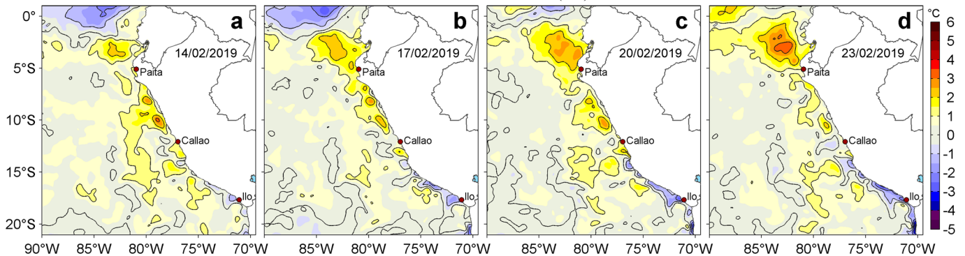
Figura 3. Anomalías de la temperatura superficial del mar (TSM, °C) para los días: a) 14, b) 17, c) 20 y d) 23 de febrero de 2019. Las anomalías se calcularon respecto de la climatología para el periodo 2007-2016. Datos: OSTIA-UKMO-L4-GLOB-v2.0 (UK Met Office, 2012; Donlon et al, 2012). Procesamiento: LHF/AFIOF/DGIOCC/IMARPE.
