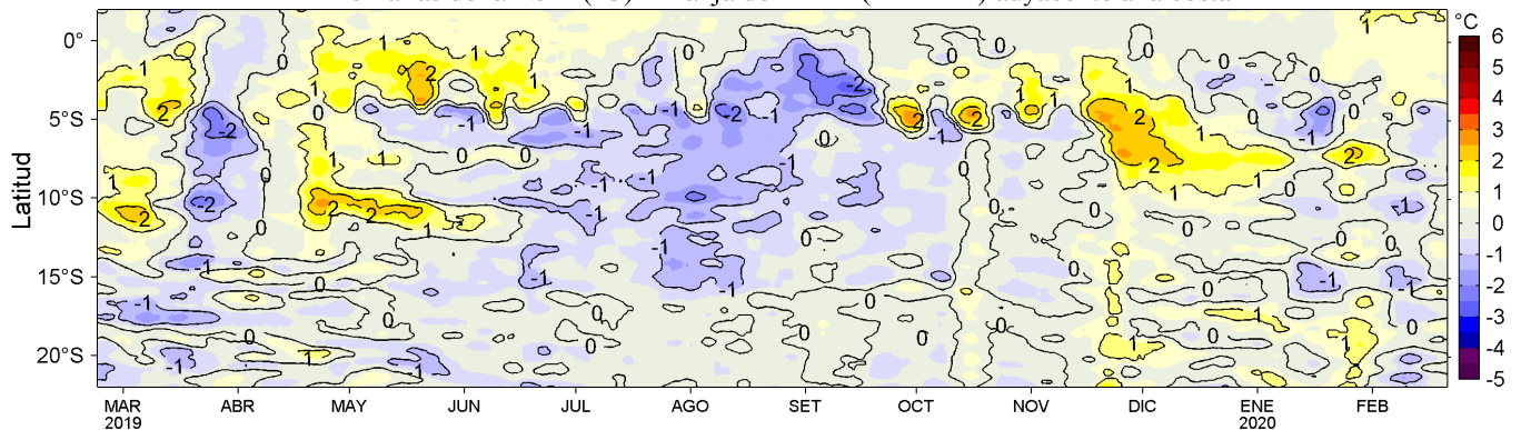
Figura 4. Variación promedio de las anomalías de la temperatura superficial del mar (TSM, °C) para una franja de 60 mn (~111 km) adyacente al litoral peruano para los últimos doce meses al 21 de febrero de 2020. Datos: OSTIA-UKMO-L4-GLOB-v2.0 (UK Met. Office, 2012; Donlon et al, 2012) disponible en https://podaac.jpl.nasa.gov/dataset/OSTIA-UKMO-L4-GLOB-v2.0 . Las anomalías se calcularon con respecto al periodo 2007-2016. Procesamiento: LHF/AFIOF/DGIOCC/IMARPE.
