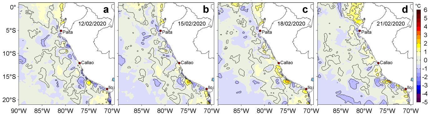
Figura 3. Anomalías de la temperatura superficial del mar (TSM, °C) para los días: a) 12, b) 15, c) 18 y d) 21 de febrero de 2020. Las anomalías se calcularon respecto de la climatología para el periodo 2007-2016. Datos: OSTIA-UKMO-L4-GLOB-v2.0 (UK Met Office, 2012; Donlon et al, 2012). Procesamiento: LHF/AFIOF/DGIOCC/IMARPE.
