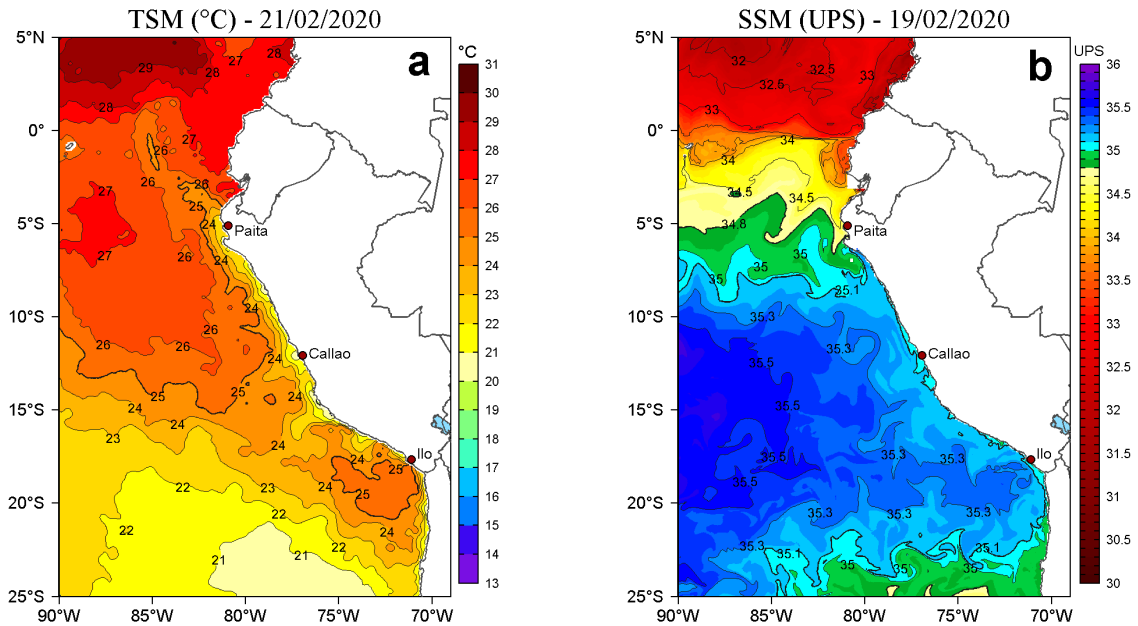
Figura 2. a) Temperatura superficial del mar (TSM, °C) y b) Salinidad superficial del mar (SSM, UPS), para el 21 y 19 de febrero de 2020, respectivamente. Datos: OSTIA-UKMO-L4-GLOB-v2.0 (UK Met Office, 2012; Donlon et al, 2012) disponible en https://podaac.jpl.nasa.gov/dataset/OSTIA-UKMO-L4-GLOB-v2.0 para (a) y Hybrid Coordinate Ocean Model v. GOF5 3.1 (HYCOM; Halliwell et al., 1998; 2000; Bleck, 2001) para (b). Procesamiento: LHF/AFIOF/DGIOCC/IMARPE.
