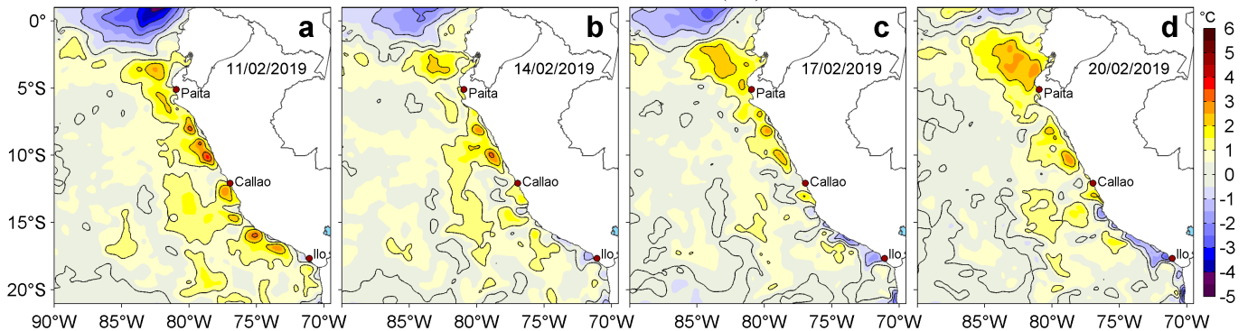
Figura 3. Anomalías de la temperatura superficial del mar (TSM, °C) para los días: a) 11, b) 14, c) 17 y d) 20 de febrero de 2019. Las anomalías se calcularon respecto de la climatología para el periodo 2007-2016. Datos: OSTIA-UKMO-L4-GLOB-v2.0 (UK Met Office, 2012; Donlon et al, 2012). Procesamiento: LHF/AFIOF/DGIOCC/IMARPE.
