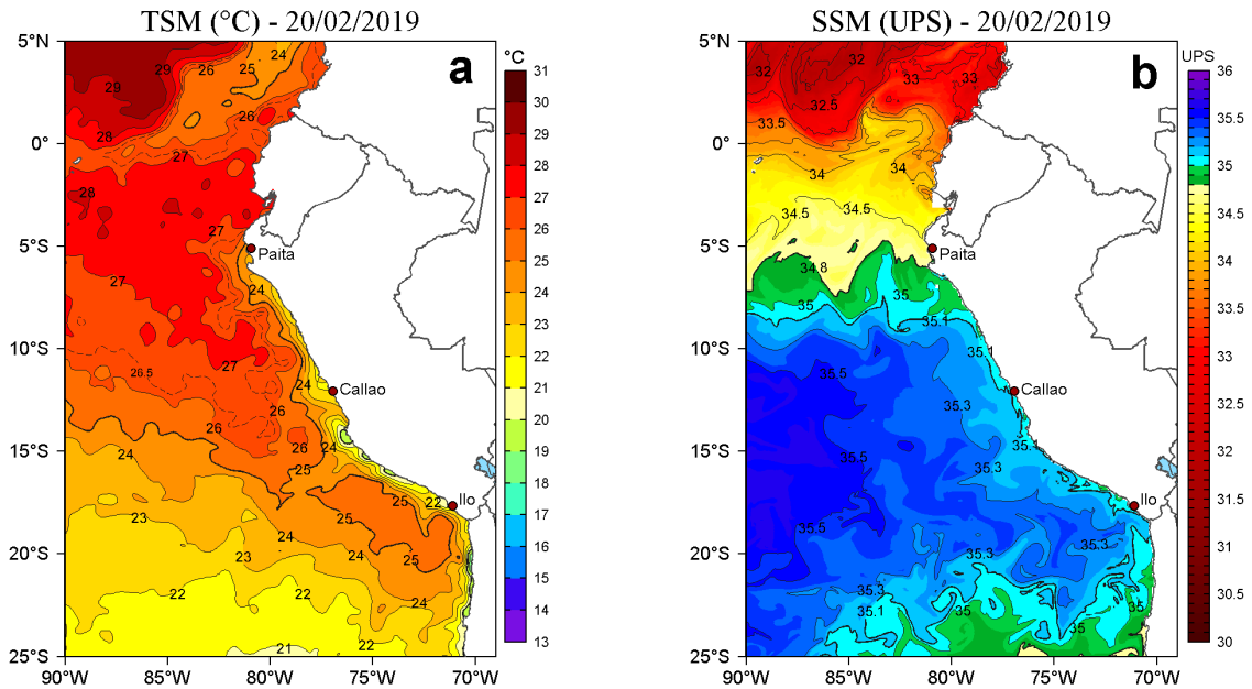
Figura 2. a) Temperatura superficial del mar (TSM, °C) y b) Salinidad superficial del mar (SSM, UPS) para el 20 de febrero de 2019. Datos: OSTIA-UKMO-L4-GLOB-v2.0 (UK Met Office, 2012; Donlon et al, 2012) disponible en https://podaac.jpl.nasa.gov/dataset/OSTIA-UKMO-L4-GLOB-v2.0 para (a) y Hybrid Coordinate Ocean Model v. GOF3 3.1 (HYCOM; Halliwell et al., 1998; 2000; Bleck, 2001) para (b). Procesamiento: LHF/AFIOF/DGIOCC/IMARPE.
