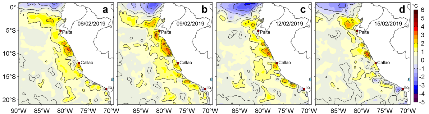
Figura 3. Anomalías de la temperatura superficial del mar (TSM, °C) para los días: a) 06, b) 09, c) 12 y d) 15 de febrero de 2019. Las anomalías se calcularon respecto de la climatología para el periodo 2007-2016. Datos: OSTIA-UKMO-L4-GLOB-v2.0 (UK Met Office, 2012; Donlon et al, 2012). Procesamiento: LHF/AFIOF/DGIOCC/IMARPE.
