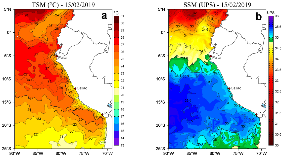
Figura 2. a) Temperatura superficial del mar (TSM, °C) y b) Salinidad superficial del mar (SSM, UPS) para el 15 de febrero de 2019. Datos: OSTIA-UKMO-L4-GLOB-v2.0 (UK Met Office, 2012; Donlon et al, 2012) disponible en https://podaac.jpl.nasa.gov/dataset/OSTIA-UKMO-L4-GLOB-v2.0 para (a) y Hybrid Coordinate Ocean Model v. GOF3 3.1 (HYCOM; Halliwell et al., 1998; 2000; Bleck, 2001) para (b). Procesamiento: LHF/AFIOF/DGIOCC/IMARPE.
