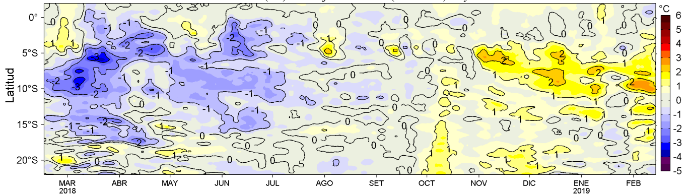
Figura 4. Variación promedio de las anomalías de la temperatura superficial del mar (TSM, °C) para una franja de 60 mn (~111 km) adyacente al litoral peruano para los últimos doce meses al 14 de febrero de 2019. Datos: OSTIA-UKMO-L4-GLOB-v2.0 (UK Met. Office, 2012; Donlon et al, 2012) disponible en https://podaac.jpl.nasa.gov/dataset/OSTIA-UKMO-L4-GLOB-v2.0 . Las anomalías se calcularon con respecto al periodo 2007-2016. Procesamiento: LHF/AFIOF/DGIOCC/IMARPE.
