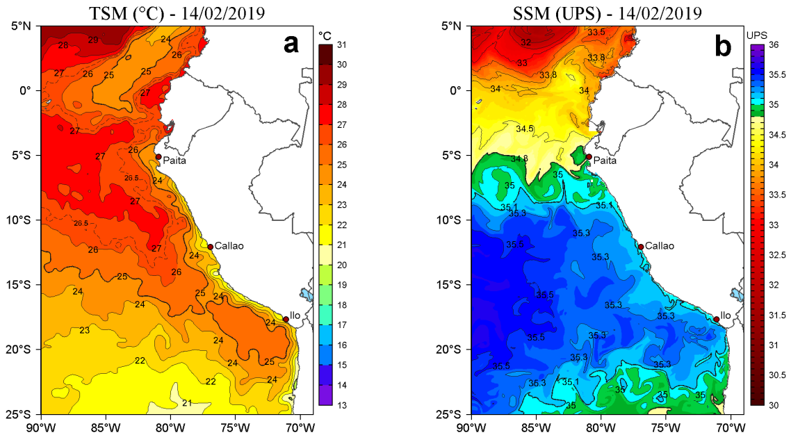
Figura 2. a) Temperatura superficial del mar (TSM, °C) y b) Salinidad superficial del mar (SSM, UPS) para el 14 de febrero de 2019. Datos: OSTIA-UKMO-L4-GLOB-v2.0 (UK Met Office, 2012; Donlon et al, 2012) disponible en https://podaac.jpl.nasa.gov/dataset/OSTIA-UKMO-L4-GLOB-v2.0 para (a) y Hybrid Coordinate Ocean Model v. GOF3 3.1 (HYCOM; Halliwell et al., 1998; 2000; Bleck, 2001) para (b). Procesamiento: LHF/AFIOF/DGIOCC/IMARPE.
