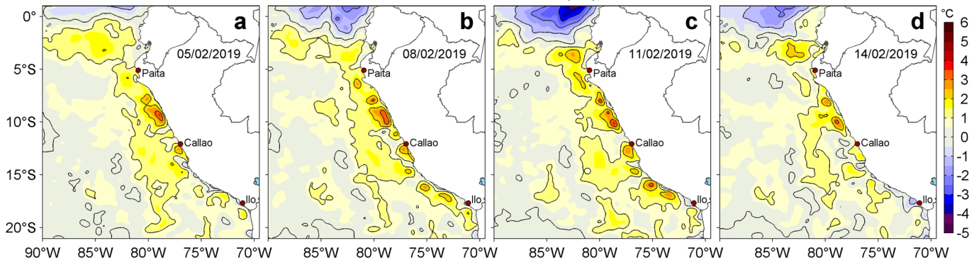
Figura 3. Anomalías de la temperatura superficial del mar (TSM, °C) para los días: a) 05, b) 08, c) 11 y d) 14 de febrero de 2019. Las anomalías se calcularon respecto de la climatología para el periodo 2007-2016. Datos: OSTIA-UKMO-L4-GLOB-v2.0 (UK Met Office, 2012; Donlon et al, 2012). Procesamiento: LHF/AFIOF/DGIOCC/IMARPE.
