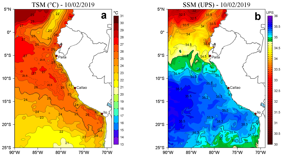
Figura 2. a) Temperatura superficial del mar (TSM, °C) y b) Salinidad superficial del mar (SSM, UPS) para el 10 de febrero de 2019. Datos: OSTIA-UKMO-L4-GLOB-v2.0 (UK Met Office, 2012; Donlon et al, 2012) disponible en https://podaac.jpl.nasa.gov/dataset/OSTIA-UKMO-L4-GLOB-v2.0 para (a) y Hybrid Coordinate Ocean Model v. GOF3 3.1 (HYCOM; Halliwell et al., 1998; 2000; Bleck, 2001) para (b). Procesamiento: LHF/AFIOF/DGIOCC/IMARPE.
