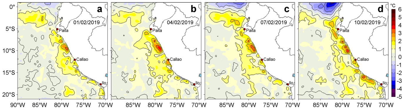
Figura 3. Anomalías de la temperatura superficial del mar (TSM, °C) para los días: a) 01, b) 04, c) 07 y d) 10 de febrero de 2019. Las anomalías se calcularon respecto de la climatología para el periodo 2007-2016. Datos: OSTIA-UKMO-L4-GLOB-v2.0 (UK Met Office, 2012; Donlon et al, 2012). Procesamiento: LHF/AFIOF/DGIOCC/IMARPE.
