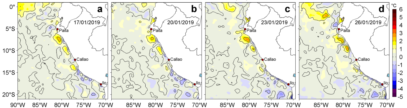
Figura 3. Anomalías de la temperatura superficial del mar (TSM, °C) para los días: a) 17, b) 20, c) 23 y d) 26 de enero de 2019. Las anomalías se calcularon respecto de la climatología para el periodo 2007-2016. Datos: OSTIA-UKMO-L4-GLOB-v2.0 (UK Met Office, 2012; Donlon et al, 2012). Procesamiento: LHF/AFIOF/DGIOCC/IMARPE.
