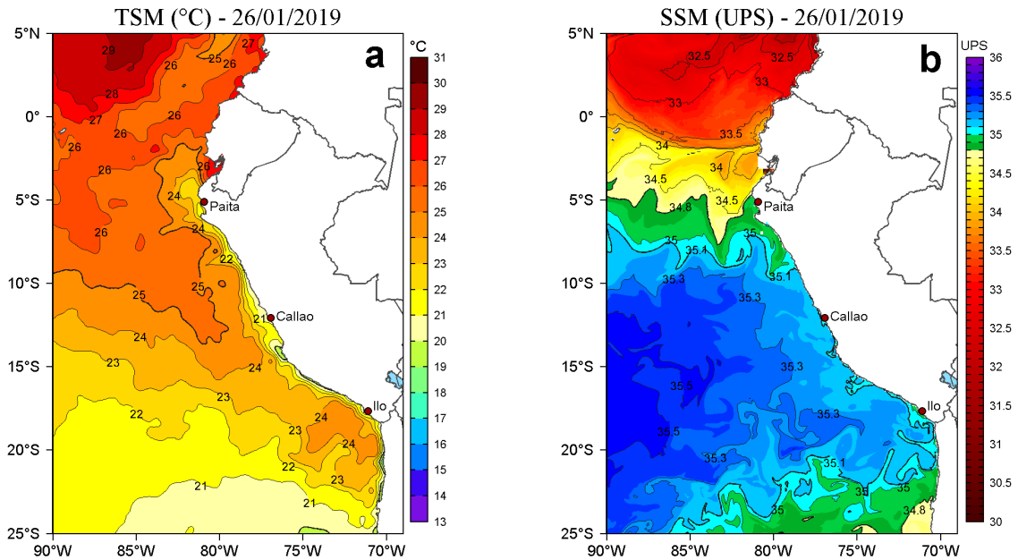
Figura 2. a) Temperatura superficial del mar (TSM, °C) y b) Salinidad superficial del mar (SSM, UPS) para el 26 de enero de 2019. Datos: OSTIA-UKMO-L4-GLOB-v2.0 (UK Met Office, 2012; Donlon et al, 2012) disponible en https://podaac.jpl.nasa.gov/dataset/OSTIA-UKMO-L4-GLOB-v2.0 para (a) y Hybrid Coordinate Ocean Model v. GOF3 3.1 (HYCOM; Halliwell et al., 1998; 2000; Bleck, 2001) para (b). Procesamiento: LHF/AFIOF/DGIOCC/IMARPE.
