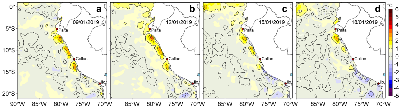
Figura 3. Anomalías de la temperatura superficial del mar (TSM, °C) para los días: a) 09, b) 12, c) 15 y d) 18 de enero de 2019. Las anomalías se calcularon respecto de la climatología para el periodo 2007-2016. Datos: OSTIA-UKMO-L4-GLOB-v2.0 (UK Met Office, 2012; Donlon et al, 2012). Procesamiento: LHFM/AFIOF/DGIOCC/IMARPE.
