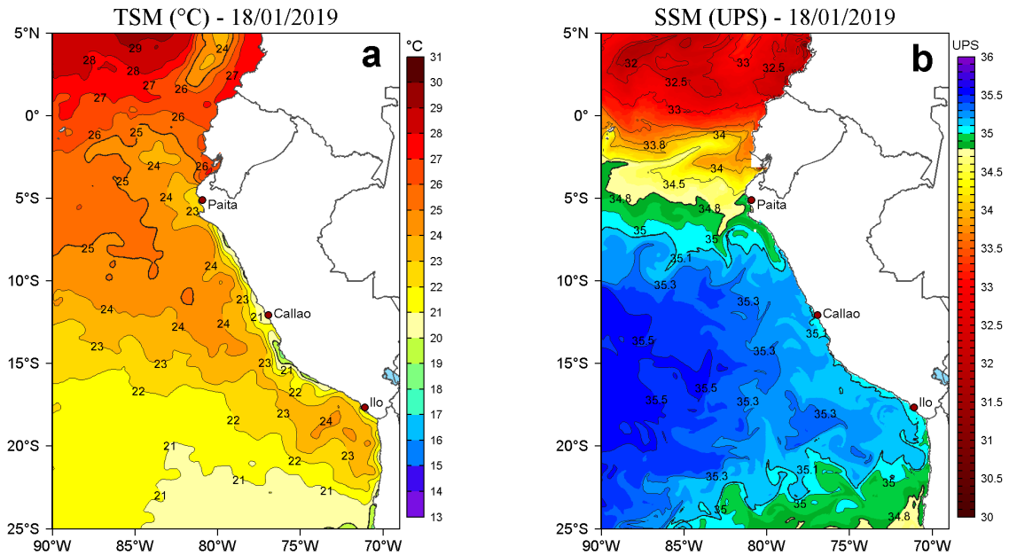
Figura 2. a) Temperatura superficial del mar (TSM, °C) y b) Salinidad superficial del mar (SSM, UPS) para el 18 de enero de 2019. Datos: OSTIA-UKMO-L4-GLOB-v2.0 (UK Met Office, 2012; Donlon et al, 2012) disponible en https://podaac.jpl.nasa.gov/dataset/OSTIA-UKMO-L4-GLOB-v2.0 para (a) y Hybrid Coordinate Ocean Model v. GOF3 3.1 (HYCOM; Halliwell et al., 1998; 2000; Bleck, 2001) para (b). Procesamiento: LHFM/AFIOF/DGIOCC/IMARPE.
