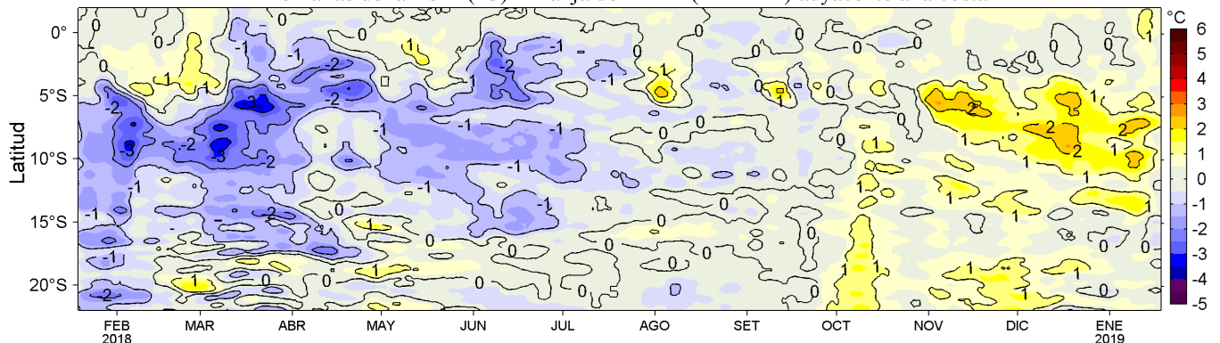
Figura 4. Variación promedio de las anomalías de la temperatura superficial del mar (TSM, °C) para una franja de 60 mn (~111 km) adyacente al litoral peruano para los últimos doce meses al 18 de enero de 2019. Datos: OSTIA-UKMO-L4-GLOB-v2.0 (UK Met. Office, 2012; Donlon et al, 2012) disponible en https://podaac.jpl.nasa.gov/dataset/OSTIA-UKMO-L4-GLOB-v2.0 . Las anomalías se calcularon con respecto al periodo 2007-2016. Procesamiento: LHFM/AFIOF/DGIOCC/IMARPE.
