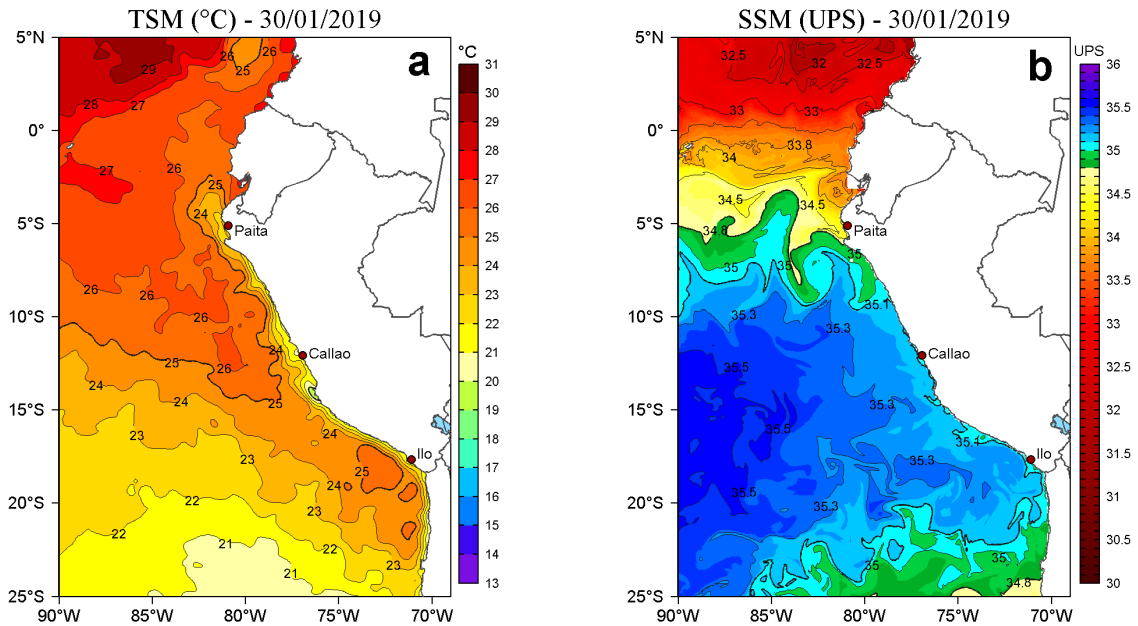
Figura 2. a) Temperatura superficial del mar (TSM, °C) y b) Salinidad superficial del mar (SSM, UPS) para el 30 de enero de 2019. Datos: OSTIA-UKMO-L4-GLOB-v2.0 (UK Met Office, 2012; Donlon et al, 2012) disponible en https://podaac.jpl.nasa.gov/dataset/OSTIA-UKMO-L4-GLOB-v2.0 para (a) y Hybrid Coordinate Ocean Model v. GOFS 3.1 (HYCOM; Halliwell et al., 1998; 2000; Bleck, 2001) para (b). Procesamiento: LHFM/AFIOF/DGIOCC/IMARPE.
