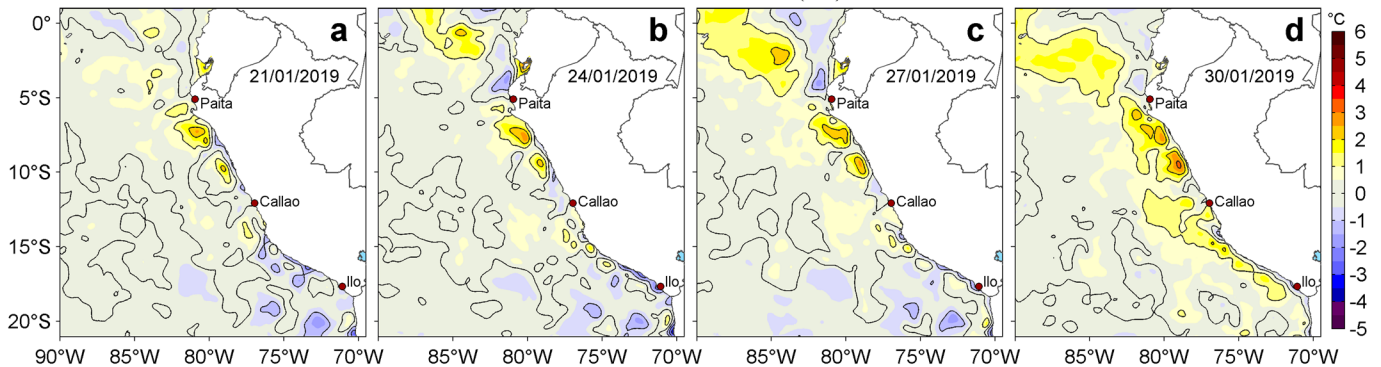
Figura 3. Anomalías de la temperatura superficial del mar (TSM, °C) para los días: a) 21, b) 24, c) 27 y d) 30 de enero de 2019. Las anomalías se calcularon respecto de la climatología para el periodo 2007-2016. Datos: OSTIA-UKMO-L4-GLOB-v2.0 (UK Met Office, 2012; Donlon et al, 2012). Procesamiento: LHFM/AFIOF/DGIOCC/IMARPE.
