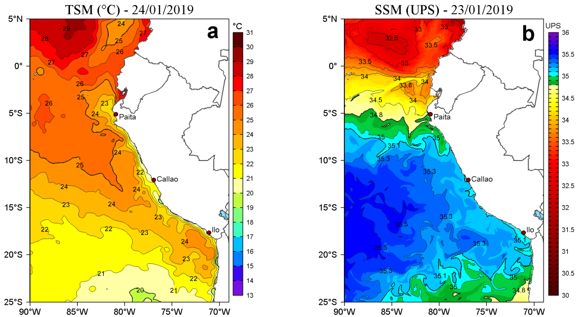
Figura 2. a) Temperatura superficial del mar (TSM, °C) para el 24 de enero de 2019 y b) Salinidad superficial del mar (SSM, UPS) para el 23 de enero de 2019. Datos: OSTIA-UKMO-L4-GLOB-v2.0 (UK Met Office, 2012; Donlon et al, 2012) disponible en https://podaac.jpl.nasa.gov/dataset/OSTIA-UKMO-L4-GLOB-v2.0 para (a) y Hybrid Coordinate Ocean Model v. GOFS 3.1 (HYCOM; Halliwell et al., 1998; 2000; Bleck, 2001) para (b). Procesamiento: LHF/AFIOF/DGIOCC/IMARPE.
