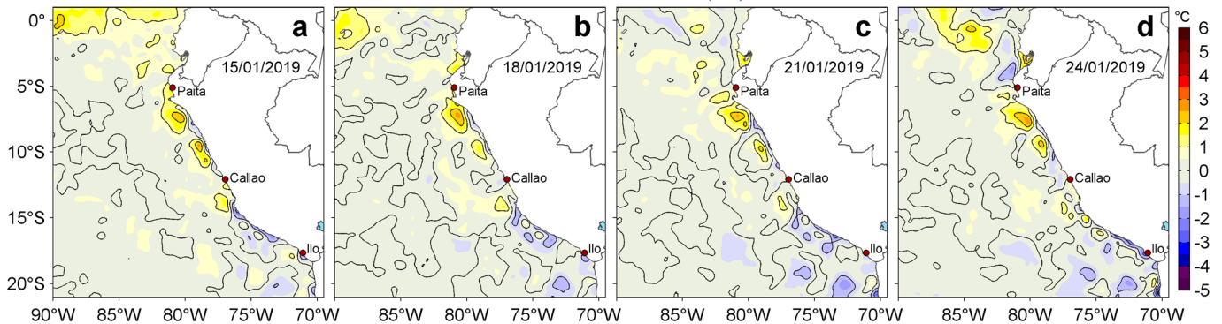
Figura 3. Anomalías de la temperatura superficial del mar (TSM, °C) para los días: a) 15, b) 18, c) 21 y d) 24 de enero de 2019. Las anomalías se calcularon respecto de la climatología para el periodo 2007-2016. Datos: OSTIA-UKMO-L4-GLOB-v2.0 (UK Met Office, 2012; Donlon et al, 2012). Procesamiento: LHF/AFIOF/DGIOCC/IMARPE.
