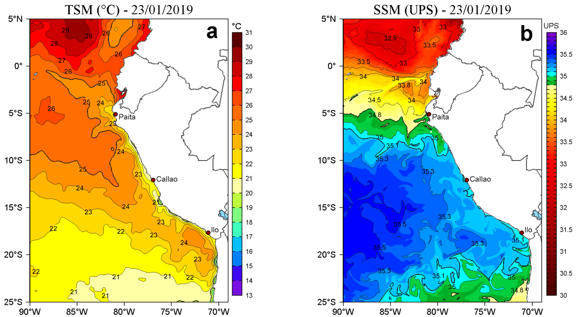
Figura 2. a) Temperatura superficial del mar (TSM, °C) y b) Salinidad superficial del mar (SSM, UPS) para el 23 de enero de 2019. Datos: OSTIA-UKMO-L4-GLOB-v2.0 (UK Met Office, 2012; Donlon et al, 2012) disponible en https://podaac.jpl.nasa.gov/dataset/OSTIA-UKMO-L4-GLOB-v2.0 para (a) y Hybrid Coordinate Ocean Model v. GOF3 3.1 (HYCOM; Halliwell et al., 1998; 2000; Bleck, 2001) para (b). Procesamiento: LHF/AFIOF/DGIOCC/IMARPE.
