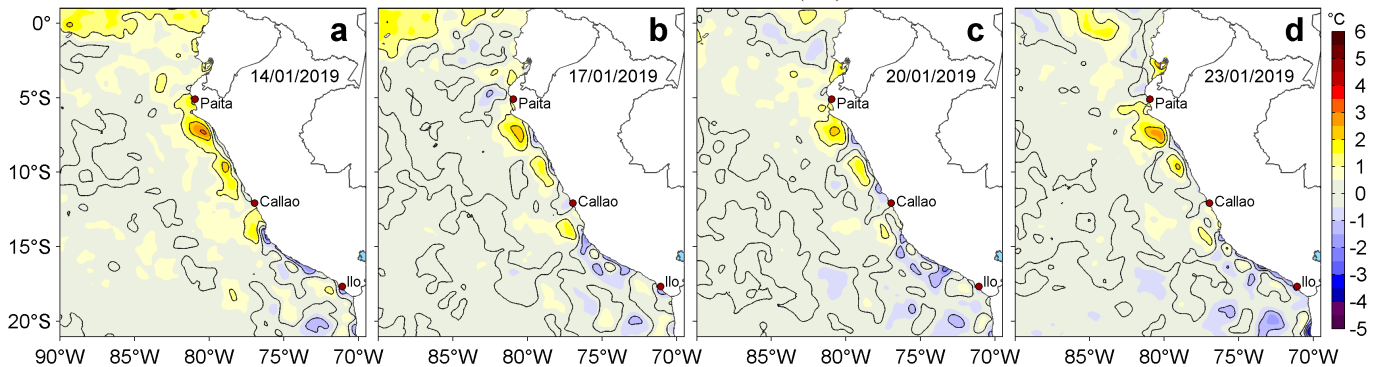
Figura 3. Anomalías de la temperatura superficial del mar (TSM, °C) para los días: a) 14, b) 17, c) 20 y d) 23 de enero de 2019. Las anomalías se calcularon respecto de la climatología para el periodo 2007-2016. Datos: OSTIA-UKMO-L4-GLOB-v2.0 (UK Met Office, 2012; Donlon et al, 2012). Procesamiento: LHF/AFIOF/DGIOCC/IMARPE.
