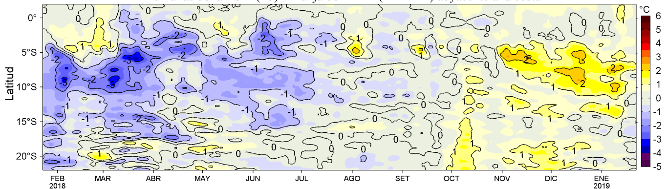
Figura 4. Variación promedio de las anomalías de la temperatura superficial del mar (TSM, °C) para una franja de 60 mn (~111 km) adyacente al litoral peruano para los últimos doce meses al 22 de enero de 2019. Datos: OSTIA-UKMO-L4-GLOB-v2.0 (UK Met. Office, 2012; Donlon et al, 2012) disponible en https://podaac.jpl.nasa.gov/dataset/OSTIA-UKMO-L4-GLOB-v2.0 . Las anomalías se calcularon con respecto al periodo 2007-2016. Procesamiento: LHFM/AFIOF/DGIOCC/IMARPE.
