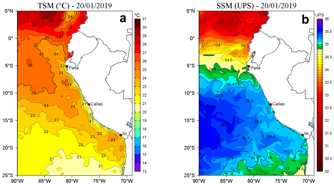
Figura 2. a) Temperatura superficial del mar (TSM, °C) y b) Salinidad superficial del mar (SSM, UPS) para el 20 de enero de 2019. Datos: OSTIA-UKMO-L4-GLOB-v2.0 (UK Met Office, 2012; Donlon et al, 2012) disponible en https://podaac.jpl.nasa.gov/dataset/OSTIA-UKMO-L4-GLOB-v2.0 para (a) y Hybrid Coordinate Ocean Model v. GOFS 3.1 (HYCOM; Halliwell et al., 1998; 2000; Bleck, 2001) para (b). Procesamiento: LHFM/AFIOF/DGIOCC/IMARPE.
