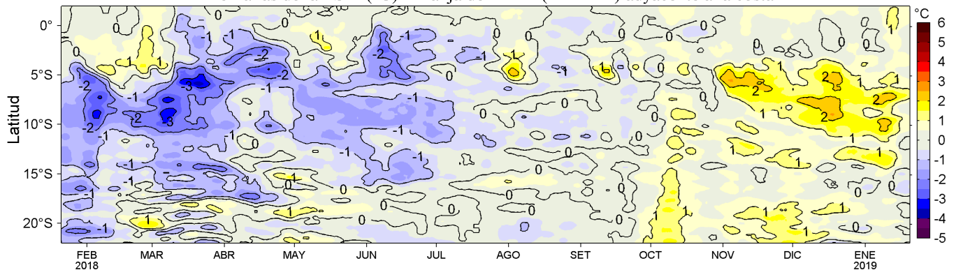
Figura 4. Variación promedio de las anomalías de la temperatura superficial del mar (TSM, °C) para una franja de 60 mn (~111 km) adyacente al litoral peruano para los últimos doce meses al 20 de enero de 2019. Datos: OSTIA-UKMO-L4-GLOB-v2.0 (UK Met. Office, 2012; Donlon et al, 2012) disponible en https://podaac.jpl.nasa.gov/dataset/OSTIA-UKMO-L4-GLOB-v2.0 . Las anomalías se calcularon con respecto al periodo 2007-2016. Procesamiento: LHFM/AFIOF/DGIOCC/IMARPE.
