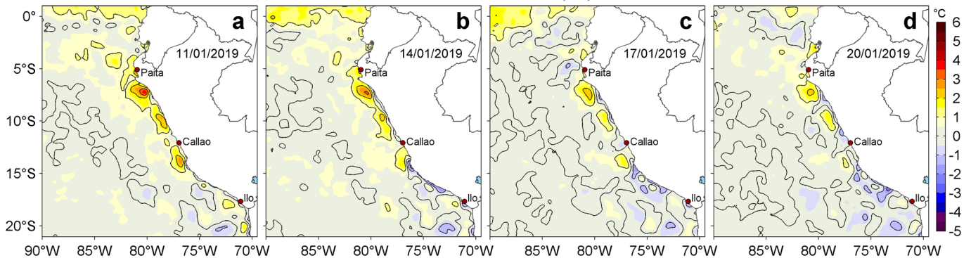
Figura 3. Anomalías de la temperatura superficial del mar (TSM, °C) para los días: a) 11, b) 14, c) 17 y d) 20 de enero de 2019. Las anomalías se calcularon respecto de la climatología para el periodo 2007-2016. Datos: OSTIA-UKMO-L4-GLOB-v2.0 (UK Met Office, 2012; Donlon et al, 2012). Procesamiento: LHFM/AFIOF/DGIOCC/IMARPE.
