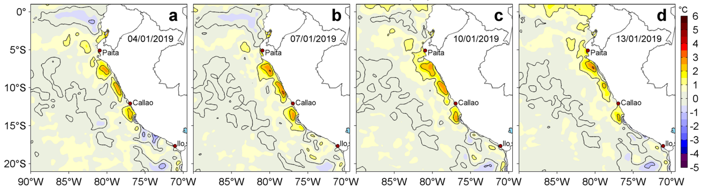
Figura 3. Anomalías de la temperatura superficial del mar (TSM, °C) para los días: a) 04, b) 07, c) 10 y d) 13 de enero de 2019. Las anomalías se calcularon respecto de la climatología para el periodo 2007-2016. Datos: OSTIA-UKMO-L4-GLOB-v2.0 (UK Met Office, 2012; Donlon et al, 2012). Procesamiento: LHF/AFIOF/DGIOCC/IMARPE.
