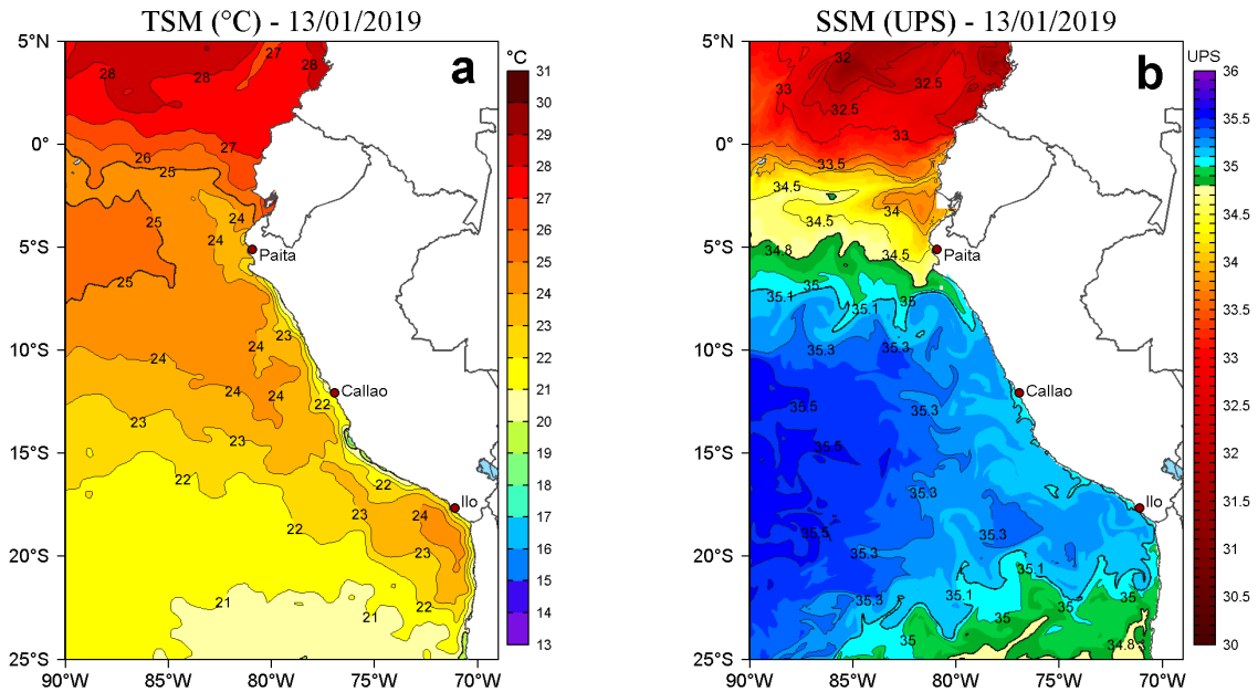
Figura 2. a) Temperatura superficial del mar (TSM, °C) y b) Salinidad superficial del mar (SSM, UPS) para el 13 de enero de 2019. Datos: OSTIA-UKMO-L4-GLOB-v2.0 (UK Met Office, 2012; Donlon et al, 2012) disponible en https://podaac.jpl.nasa.gov/dataset/OSTIA-UKMO-L4-GLOB-v2.0 para (a) y Hybrid Coordinate Ocean Model v. GOF3 3.1 (HYCOM; Halliwell et al., 1998; 2000; Bleck, 2001) para (b). Procesamiento: LHF/AFIOF/DGIOCC/IMARPE.
