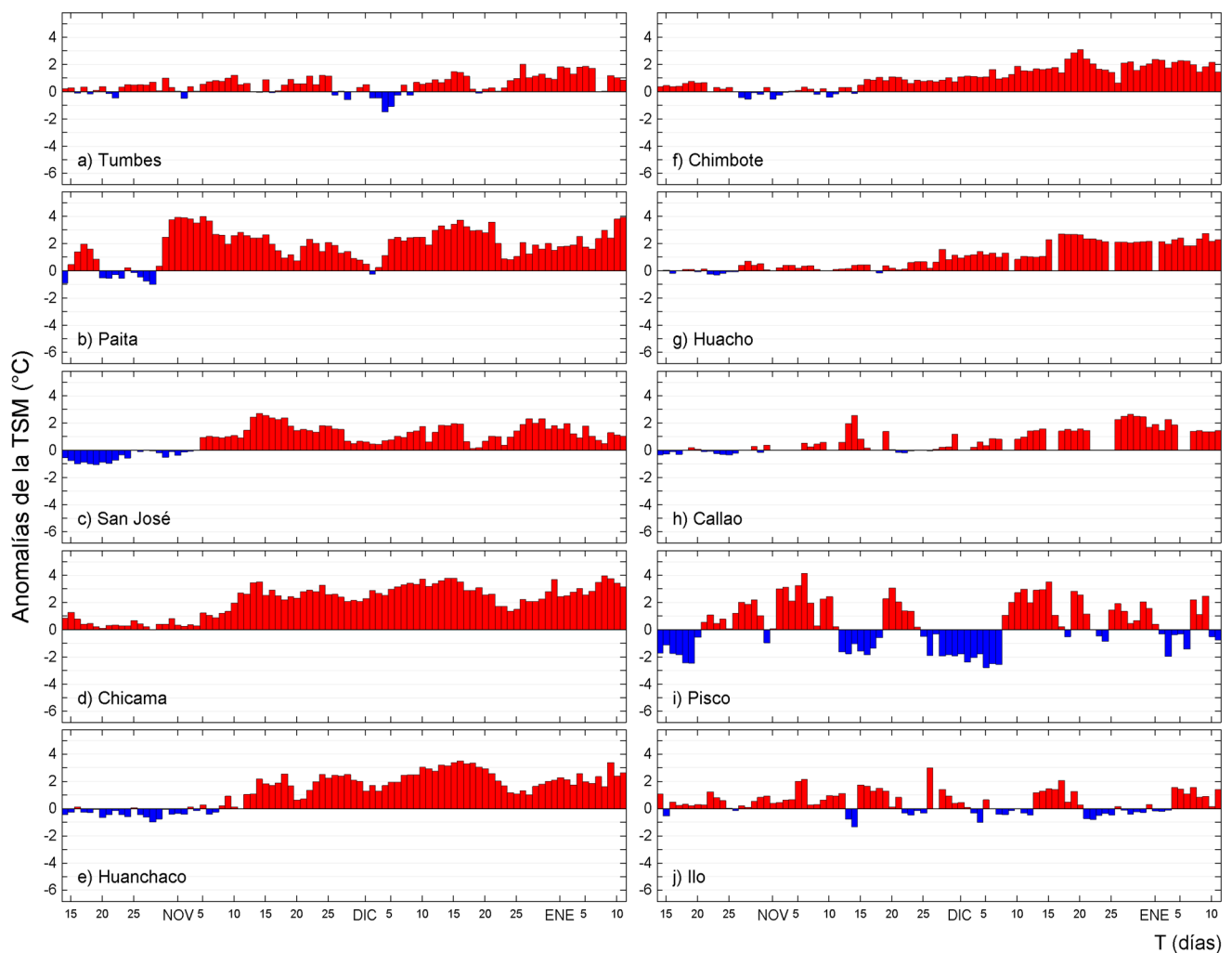
Figura 5. Variación del promedio diario de las anomalías de la temperatura superficial del mar (TSM, °C) en la red de estaciones costeras que administra IMARPE en el litoral peruano durante el último trimestre. Las anomalías se calcularon respecto del promedio climatológico pentadal (5 días) para el periodo que se indica en la Tabla 1. Datos y procesamiento: LHFM/AFIOF/DGIOCC/IMARPE.
