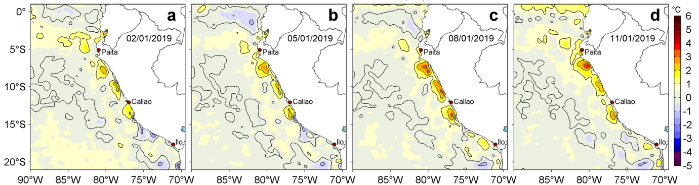
Figura 3. Anomalías de la temperatura superficial del mar (TSM, °C) para los días: a) 02, b) 05, c) 08 y d) 11 de enero de 2019. Las anomalías se calcularon respecto de la climatología para el periodo 2007-2016. Datos: OSTIA-UKMO-L4-GLOB-v2.0 (UK Met Office, 2012; Donlon et al, 2012). Procesamiento: LHF/AFIOF/DGIOCC/IMARPE.
