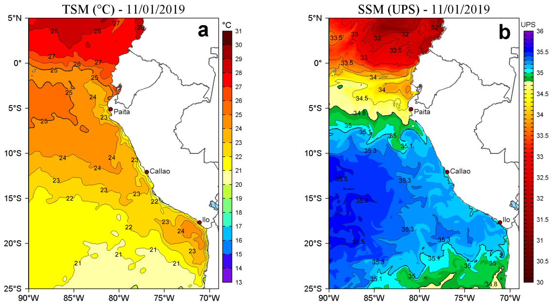
Figura 2. a) Temperatura superficial del mar (TSM, °C) y b) Salinidad superficial del mar (SSM, UPS) para el 11 de enero de 2019. Datos: OSTIA-UKMO-L4-GLOB-v2.0 (UK Met Office, 2012; Donlon et al, 2012) disponible en https://podaac.jpl.nasa.gov/dataset/OSTIA-UKMO-L4-GLOB-v2.0 para (a) y Hybrid Coordinate Ocean Model v. GOFS 3.1 (HYCOM; Halliwell et al., 1998; 2000; Bleck, 2001) para (b). Procesamiento: LHF/AFIOF/DGIOCC/IMARPE.
