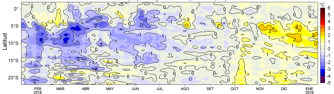
Figura 4. Variación promedio de las anomalías de la temperatura superficial del mar (TSM, °C) para una franja de 60 mn (~111 km) adyacente al litoral peruano para los últimos doce meses al 11 de enero de 2019. Datos: OSTIA-UKMO-L4-GLOB-v2.0 (UK Met. Office, 2012; Donlon et al, 2012) disponible en https://podaac.jpl.nasa.gov/dataset/OSTIA-UKMO-L4-GLOB-v2.0 . Las anomalías se calcularon con respecto al periodo 2007-2016. Procesamiento: LHF/AFIOF/DGIOCC/IMARPE.
