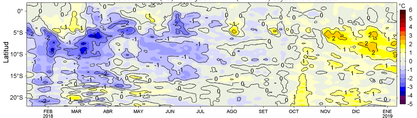
Figura 4. Variación promedio de las anomalías de la temperatura superficial del mar (TSM, °C) para una franja de 60 mn (~111 km) adyacente al litoral peruano para los últimos doce meses al 10 de enero de 2019. Datos: OSTIA-UKMO-L4-GLOB-v2.0 (UK Met. Office, 2012; Donlon et al, 2012) disponible en https://podaac.jpl.nasa.gov/dataset/OSTIA-UKMO-L4-GLOB-v2.0 . Las anomalías se calcularon con respecto al periodo 2007-2016. Procesamiento: LHF/AFIOF/DGIOCC/IMARPE.
