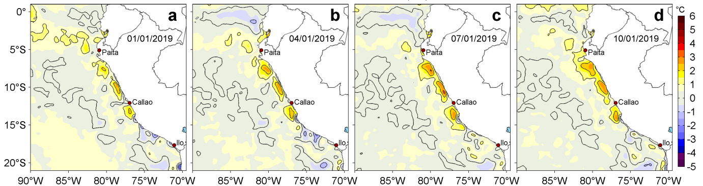
Figura 3. Anomalías de la temperatura superficial del mar (TSM, °C) para los días: a) 01, b) 04, c) 07 y d) 10 de enero de 2019. Las anomalías se calcularon respecto de la climatología para el periodo 2007-2016. Datos: OSTIA-UKMO-L4-GLOB-v2.0 (UK Met Office, 2012; Donlon et al, 2012). Procesamiento: LHF/AFIOF/DGIOCC/IMARPE.
