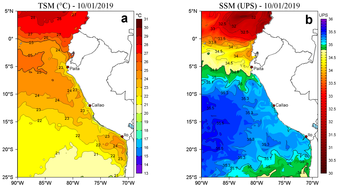
Figura 2. a) Temperatura superficial del mar (TSM, °C) y b) Salinidad superficial del mar (SSM, UPS) para el 10 de enero de 2019. Datos: OSTIA-UKMO-L4-GLOB-v2.0 (UK Met Office, 2012; Donlon et al, 2012) disponible en https://podaac.jpl.nasa.gov/dataset/OSTIA-UKMO-L4-GLOB-v2.0 para (a) y Hybrid Coordinate Ocean Model v. GOF5 3.1 (HYCOM; Halliwell et al., 1998; 2000; Bleck, 2001) para (b). Procesamiento: LHF/AFIOF/DGIOCC/IMARPE.
