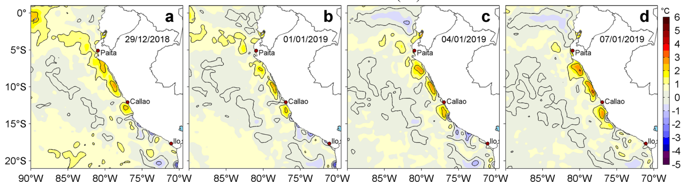
Figura 3. Anomalías de la temperatura superficial del mar (TSM, °C) para los días: a) 29 de diciembre del 2018, b) 01, c) 04 y d) 07 de enero de 2019. Las anomalías se calcularon respecto de la climatología para el periodo 2007-2016. Datos: OSTIA-UKMO-L4-GLOB-v2.0 (UK Met Office, 2012; Donlon et al, 2012). Procesamiento: LHFM/AFIOF/DGIOCC/IMARPE.
