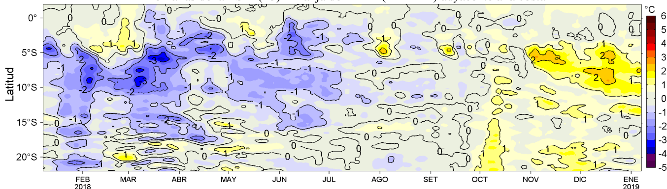
Figura 4. Variación promedio de las anomalías de la temperatura superficial del mar (TSM, °C) para una franja de 60 mn (~111 km) adyacente al litoral peruano para los últimos doce meses al 07 de enero de 2019. Datos: OSTIA-UKMO-L4-GLOB-v2.0 (UK Met. Office, 2012; Donlon et al, 2012) disponible en https://podaac.jpl.nasa.gov/dataset/OSTIA-UKMO-L4-GLOB-v2.0 . Las anomalías se calcularon con respecto al periodo 2007-2016. Procesamiento: LHFM/AFIOF/DGIOCC/IMARPE.
