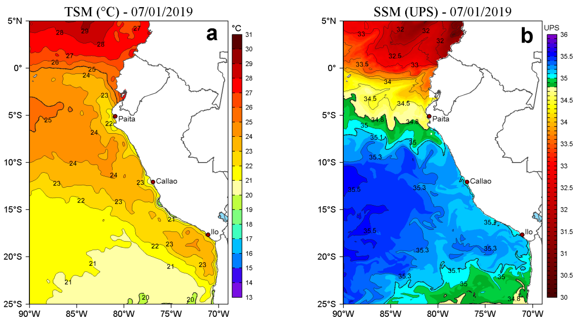
Figura 2. a) Temperatura superficial del mar (TSM, °C) y b) Salinidad superficial del mar (SSM, UPS) para el 07 de enero de 2019. Datos: OSTIA-UKMO-L4-GLOB-v2.0 (UK Met Office, 2012; Donlon et al, 2012) disponible en https://podaac.jpl.nasa.gov/dataset/OSTIA-UKMO-L4-GLOB-v2.0 para (a) y Hybrid Coordinate Ocean Model v. GOFS 3.1 (HYCOM; Halliwell et al., 1998; 2000; Bleck, 2001) para (b). Procesamiento: LHFM/AFIOF/DGIOCC/IMARPE.
