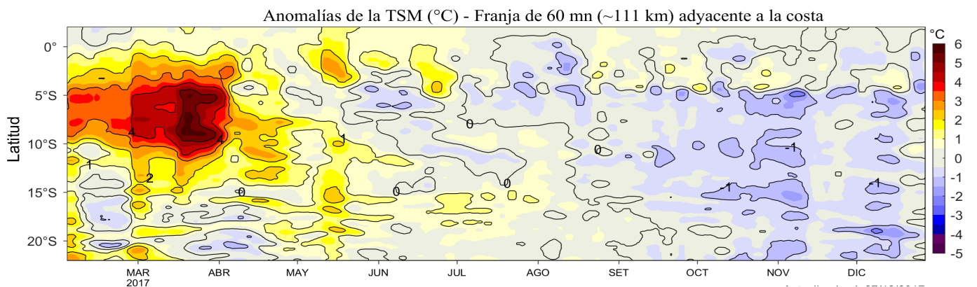
Figura 4. Variación promedio de las anomalías de la temperatura superficial del mar ( ^{\circ}\text{C} ) para una franja de 60 mn ( \sim 111 km) adyacente a la costa para los últimos doce meses al 27 de diciembre de 2017. Datos: OSTIA-UKMO-L4-GLOB-v2.0 (UK Met Office, 2012; Donlon et al, 2012) disponible en https://podaac.jpl.nasa.gov/dataset/OSTIA-UKMO-L4-GLOB-v2.0 . Las anomalías se calcularon con respecto al periodo 2007-2016. Procesamiento: LHF/AFIOF/DGIOCC/IMARPE.
