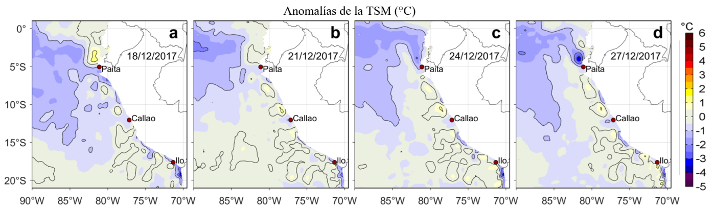
Figura 3. Anomalías de la Temperatura Superficial del Mar ( ^{\circ}\text{C} ) para los días: a) 18, b) 21, c) 24 y d) 27 de diciembre de 2017. Las anomalías se calcularon respecto de la climatología para el periodo 2007-2016. Datos: OSTIA-UKMO-L4-GLOB-v2.0 (UK Met Office, 2012; Donlon et al, 2012). Procesamiento: LHF/AFIOF/DGIOCC/IMARPE.
