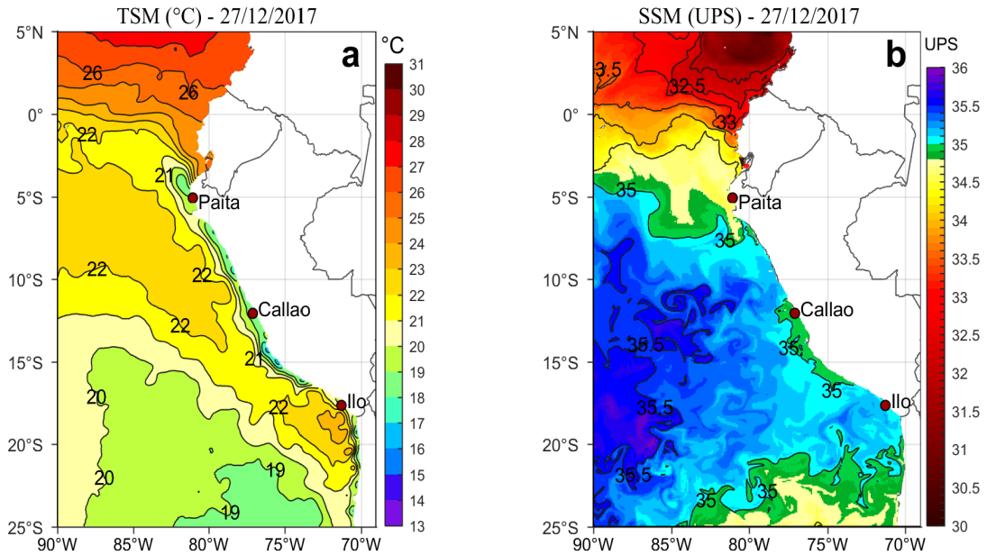
Figura 2. a) Temperatura superficial del mar ( ^{\circ}\text{C} ) y b) Salinidad superficial del mar (UPS) para el 27 de diciembre. Datos: OSTIA-UKMO-L4-GLOB-v2.0 (UK Met Office, 2012; Donlon et al, 2012) disponible en https://podaac.jpl.nasa.gov/dataset/OSTIA-UKMO-L4-GLOB-v2.0 para (a) y Hybrid Coordinate Ocean Model (HYCOM; Halliwell et al., 1998; 2000; Bleck, 2001) para (b). Procesamiento: LHF/AFIOF/DGIOCC/IMARPE.
