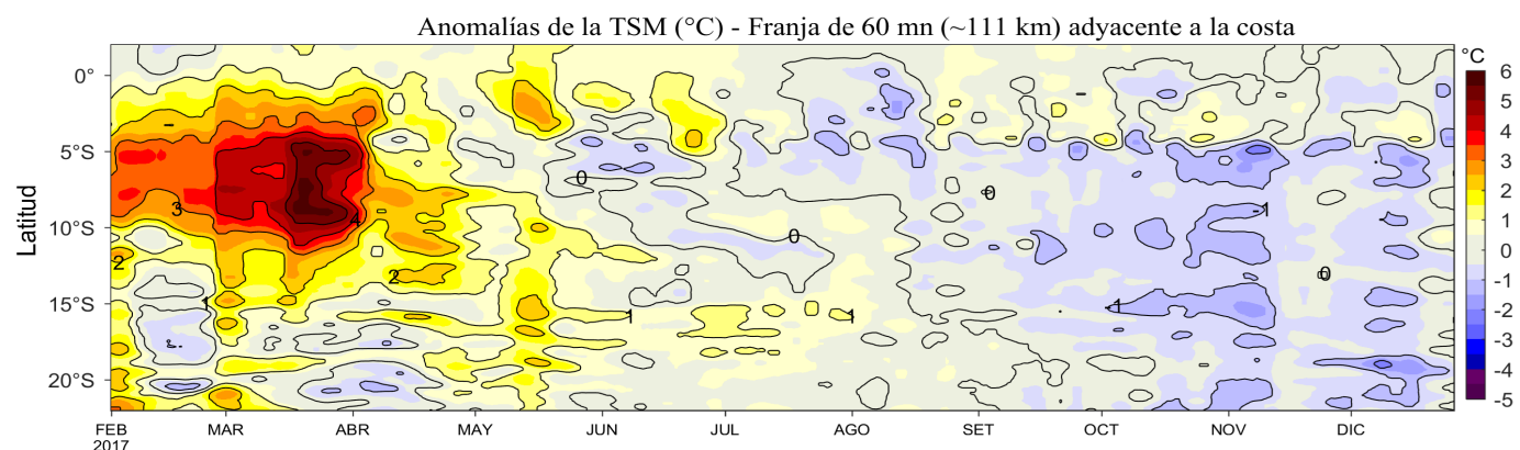
Figura 4. Variación promedio de las anomalías de la temperatura superficial del mar (°C) para una franja de 60 mn (~111 km) adyacente a la costa para los últimos doce meses al 26 de diciembre de 2017. Datos: OSTIA-UKMO-L4-GLOB-v2.0 (UK Met Office, 2012; Donlon et al, 2012) disponible en https://podaac.jpl.nasa.gov/dataset/OSTIA-UKMO-L4-GLOB-v2.0 . Las anomalías se calcularon con respecto al periodo 2007-2016. Procesamiento: LHF/AFIOF/DGIOCC/IMARPE.
