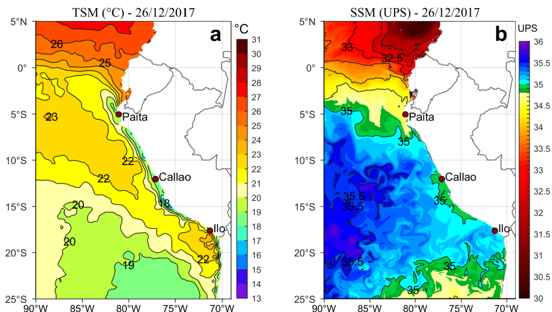
Figura 2. a) Temperatura superficial del mar (°C) y b) Salinidad superficial del mar (UPS) para el 26 de diciembre. Datos: OSTIA-UKMO-L4-GLOB-v2.0 (UK Met Office, 2012; Donlon et al, 2012) disponible en https://podaac.jpl.nasa.gov/dataset/OSTIA-UKMO-L4-GLOB-v2.0 para (a) y Hybrid Coordinate Ocean Model (HYCOM; Halliwell et al., 1998; 2000; Bleck, 2001) para (b). Procesamiento: LHF/AFIOF/DGIOCC/IMARPE.
