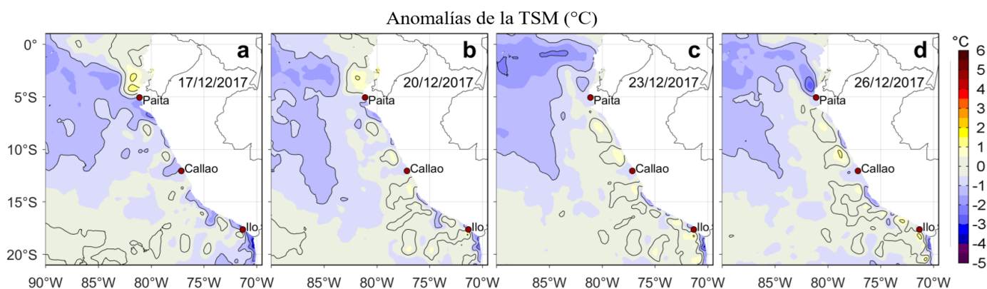
Figura 3. Anomalías de la Temperatura Superficial del Mar (°C) para los días: a) 17, b) 20, c) 23 y d) 26 de diciembre de 2017. Las anomalías se calcularon respecto de la climatología para el periodo 2007-2016. Datos: OSTIA-UKMO-L4-GLOB-v2.0 (UK Met Office, 2012; Donlon et al, 2012). Procesamiento: LHF/AFIOF/DGIOCC/IMARPE.
