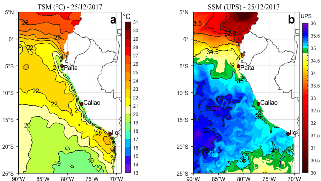
Figura 2. a) Temperatura superficial del mar (°C) y b) Salinidad superficial del mar (UPS) para el 25 de diciembre. Datos: OSTIA-UKMO-L4-GLOB-v2.0 (UK Met Office, 2012; Donlon et al, 2012) disponible en https://podaac.jpl.nasa.gov/dataset/OSTIA-UKMO-L4-GLOB-v2.0 para (a) y Hybrid Coordinate Ocean Model (HYCOM; Halliwell et al., 1998; 2000; Bleck, 2001) para (b). Procesamiento: LHF/AFIOF/DGIOCC/IMARPE.
