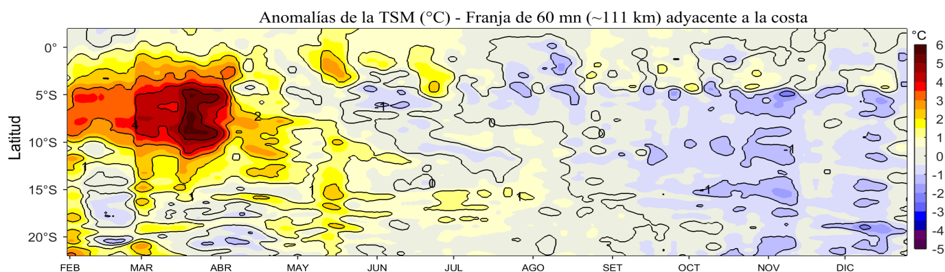
Figura 4. Variación promedio de las anomalías de la temperatura superficial del mar (°C) para una franja de 60 mn (~111 km) adyacente al litoral peruano para los últimos doce meses al 21 de diciembre de 2017. Datos: OSTIA-UKMO-L4-GLOB-v2.0 (UK Met. Office, 2012; Donlon et al, 2012) disponible en https://podaac.jpl.nasa.gov/dataset/OSTIA-UKMO-L4-GLOB-v2.0 . Las anomalías se calcularon con respecto al periodo 2007-2016. Procesamiento: LHF/AFIOF/DGIOCC/IMARPE.
