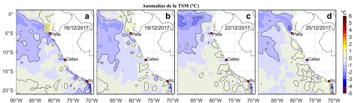
Figura 3. Anomalías de la Temperatura Superficial del Mar (°C) para los días: a) 16, b) 19, c) 22 y d) 25 de diciembre de 2017. Las anomalías se calcularon respecto de la climatología para el periodo 2007-2016. Datos: OSTIA-UKMO-L4-GLOB-v2.0 (UK Met Office, 2012; Donlon et al, 2012). Procesamiento: LHF/AFIOF/DGIOCC/IMARPE.
