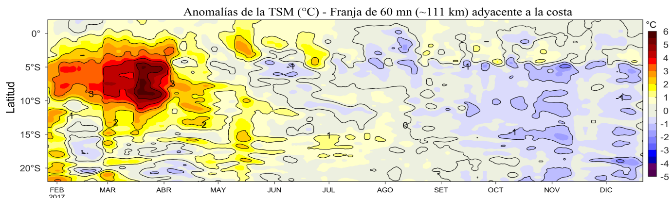
Figura 4. Variación promedio de las anomalías de la temperatura superficial del mar (°C) para una franja de 60 mn (~111 km) adyacente a la costa para los últimos doce meses al 21 de diciembre de 2017. Datos: OSTIA-UKMO-L4-GLOB-v2.0 (UK Met. Office, 2012; Donlon et al, 2012) disponible en https://podaac.jpl.nasa.gov/dataset/OSTIA-UKMO-L4-GLOB-v2.0 . Las anomalías se calcularon con respecto al periodo 2007-2016. Procesamiento: LHF/AFIOF/DGIOCC/IMARPE.
