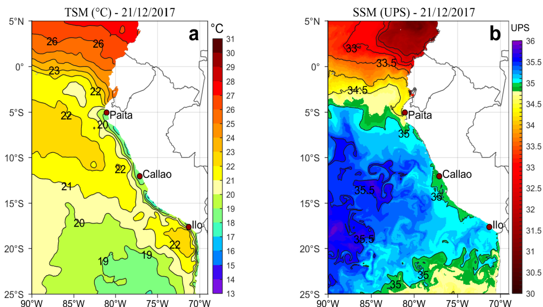
Figura 2. a) Temperatura superficial del mar (°C) y b) Salinidad superficial del mar (UPS) para el 21 de diciembre. Datos: OSTIA-UKMO-L4-GLOB-v2.0 (UK Met Office, 2012; Donlon et al, 2012) disponible en https://podaac.jpl.nasa.gov/dataset/OSTIA-UKMO-L4-GLOB-v2.0 para (a) y Hybrid Coordinate Ocean Model (HYCOM; Halliwell et al., 1998; 2000; Bleck, 2001) para (b). Procesamiento: LHF/AFIOF/DGIOCC/IMARPE.
