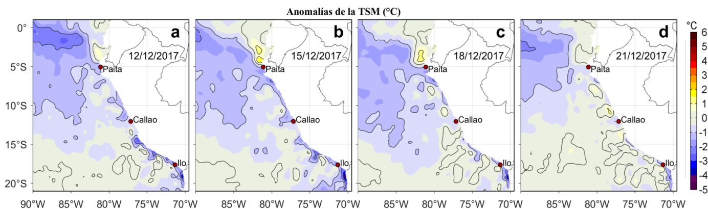
Figura 3. Anomalías de la Temperatura Superficial del Mar (°C) para los días: a) 12, b) 15, c) 18 y d) 21 de diciembre de 2017. Las anomalías se calcularon respecto de la climatología para el periodo 2007-2016. Datos: OSTIA-UKMO-L4-GLOB-v2.0 (UK Met Office, 2012; Donlon et al, 2012). Procesamiento: LHF/AFIOF/DGIOCC/IMARPE.
