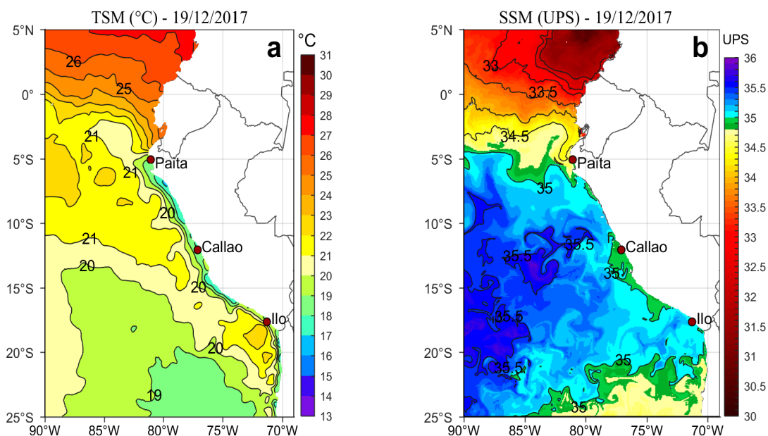
Figura 2. a) Temperatura superficial del mar (°C) y b) Salinidad superficial del mar (UPS) para el 19 de diciembre. Datos: OSTIA-UKMO-L4-GLOB-v2.0 (UK Met Office, 2012; Donlon et al, 2012) disponible en https://podaac.jpl.nasa.gov/dataset/OSTIA-UKMO-L4-GLOB-v2.0 para (a) y Hybrid Coordinate Ocean Model (HYCOM; Halliwell et al., 1998; 2000; Bleck, 2001) para (b). Procesamiento: LHF/AFIOF/DGIOCC/IMARPE.
