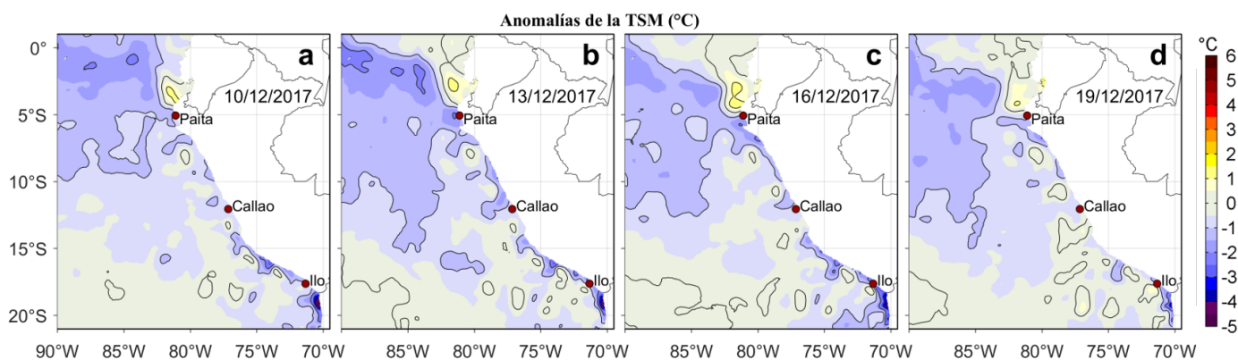
Figura 3. Anomalías de la Temperatura Superficial del Mar (°C) para los días: a) 10, b) 13, c) 16 y d) 19 de diciembre de 2017. Las anomalías se calcularon respecto de la climatología para el periodo 2007-2016. Datos: OSTIA-UKMO-L4-GLOB-v2.0 (UK Met Office, 2012; Donlon et al, 2012). Procesamiento: LHF/AFIOF/DGIOCC/IMARPE.
