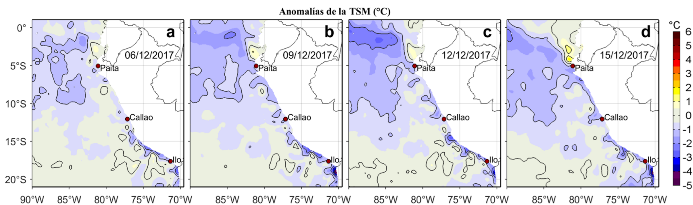
Figura 3. Anomalías de la Temperatura Superficial del Mar ( ^{\circ}\text{C} ) para los días: a) 06, b) 09, c) 12 y d) 15 de diciembre de 2017. Las anomalías se calcularon respecto de la climatología para el periodo 2007-2016. Datos: OSTIA-UKMO-L4-GLOB-v2.0 (UK Met Office, 2012; Donlon et al, 2012). Procesamiento: LHF/AFIOF/DGIOCC/IMARPE.
