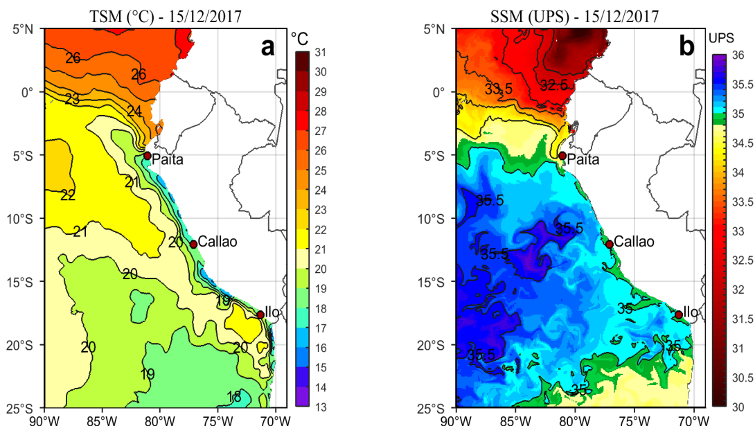
Figura 2. a) Temperatura superficial del mar ( ^{\circ}\text{C} ) y b) Salinidad superficial del mar (UPS) para el 15 de diciembre. Datos: OSTIA-UKMO-L4-GLOB-v2.0 (UK Met Office, 2012; Donlon et al, 2012) disponible en https://podaac.jpl.nasa.gov/dataset/OSTIA-UKMO-L4-GLOB-v2.0 para (a) y Hybrid Coordinate Ocean Model (HYCOM; Halliwell et al., 1998; 2000; Bleck, 2001) para (b). Procesamiento: LHF/AFIOF/DGIOCC/IMARPE.
